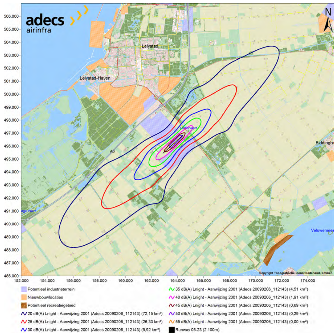
Figuur 26 20 t/m 55 dB(A) L_{\text{night}} -contouren behorende bij het referentie alternatief (Aanwijzing 2001)
