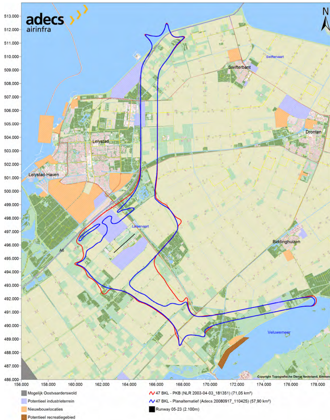
Figuur 27 47 Bkl-contour behorende bij het planalternatief.
