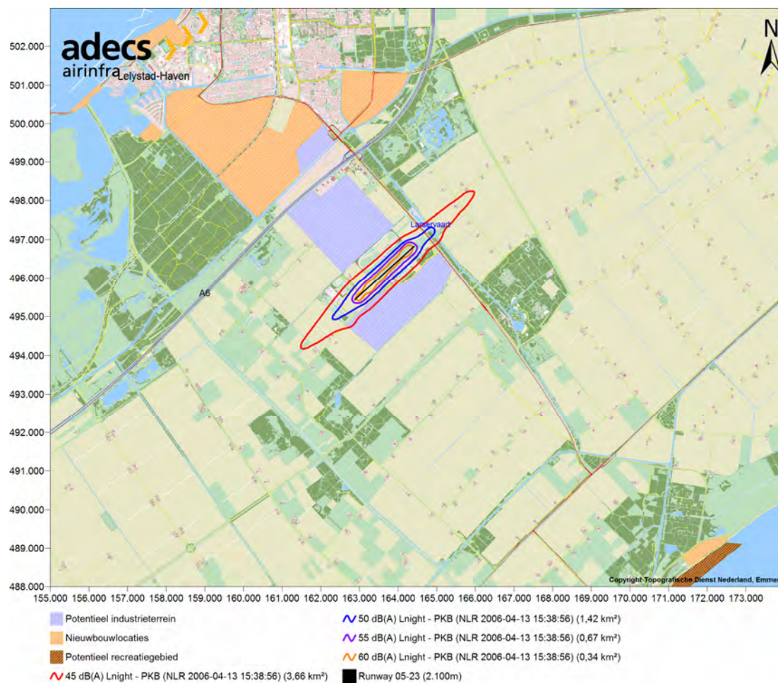
Figuur 52 45 dB(A) t/m 60 dB(A) L_{\text{night}} -contouren behorende bij de PKB.
