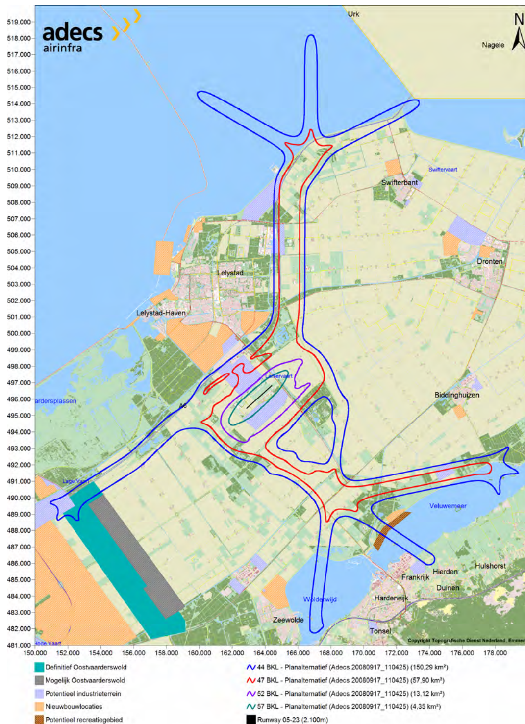
Figuur 28 44, 47, 52 en 57 Bkl-contouren behorende bij het planalternatief.
