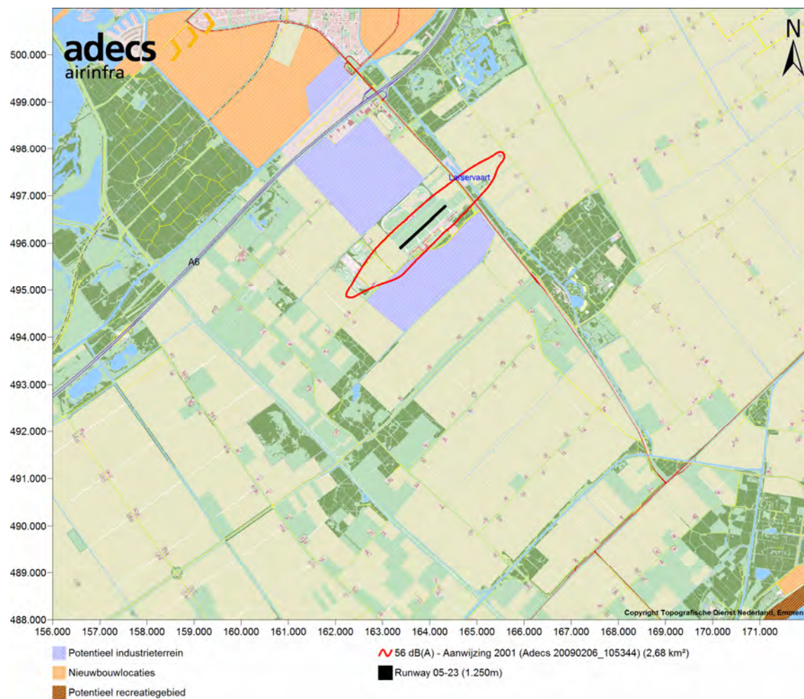
Figuur 24 56 dB(A) ) L_{den} -contour behorende bij het referentiealternatief (Aanwijzing 2001).
