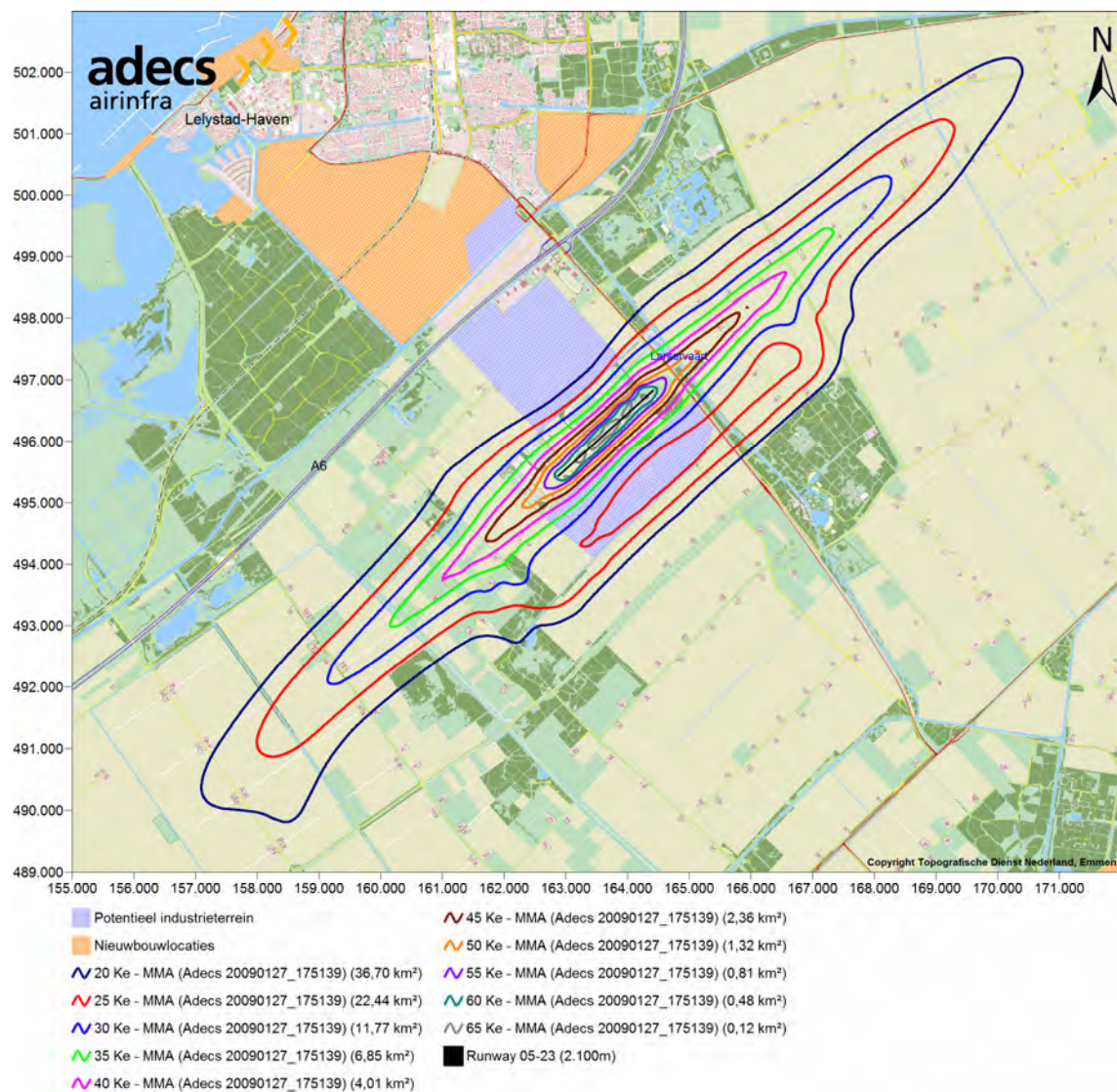
Figuur 41 20 t/m 60 Ke-contouren behorende bij het meest milieuvriendelijke alternatief.
