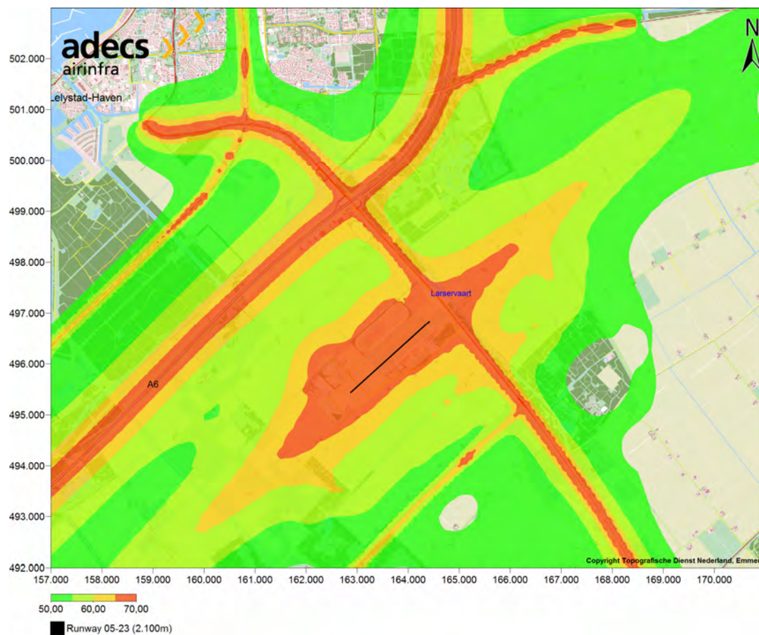
Figuur 53 Resulterende cumulatie van geluid in dB(A) voor het planalternatief (zichtjaar 2015).
