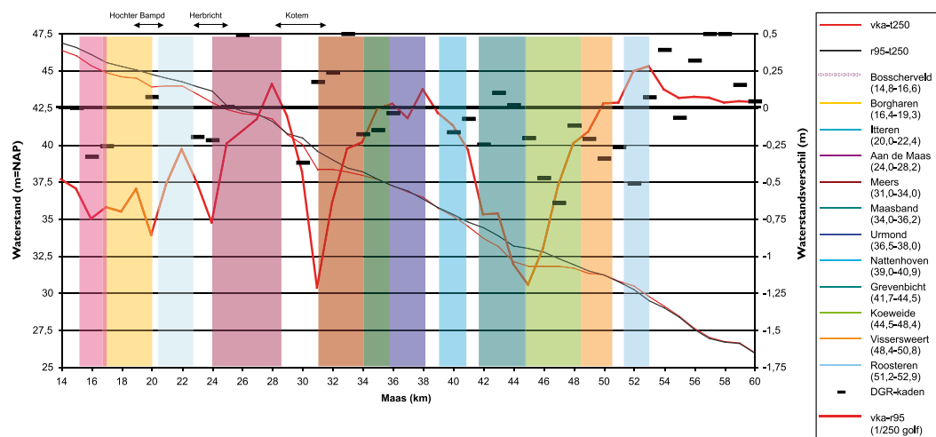
Figuur 6.1. Effect van ingrepen Voorkeursalternatief 2003: waterstanden t.o.v. referentiesituatie bij een 1:250 hoogwatergolf.
