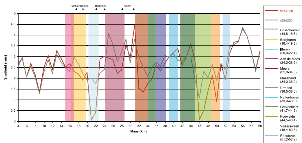
Figuur 6.2. Effect van ingrepen Voorkeursalternatief 2003: stroomsnelheden t.o.v. referentiesituatie bij een 1:250 hoogwatergolf.
