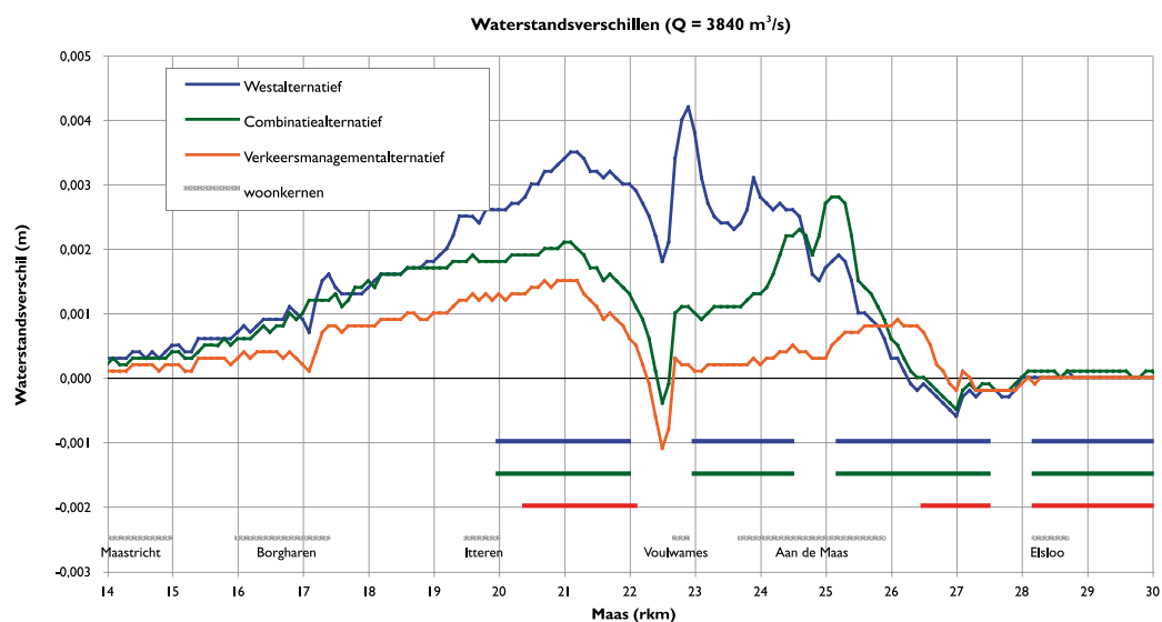
Figuur 6.3. Waterstandsverschillen van de westwaartse alternatieven ten opzichte van de referentie bij een 1:1.250 hoogwatergolf.
