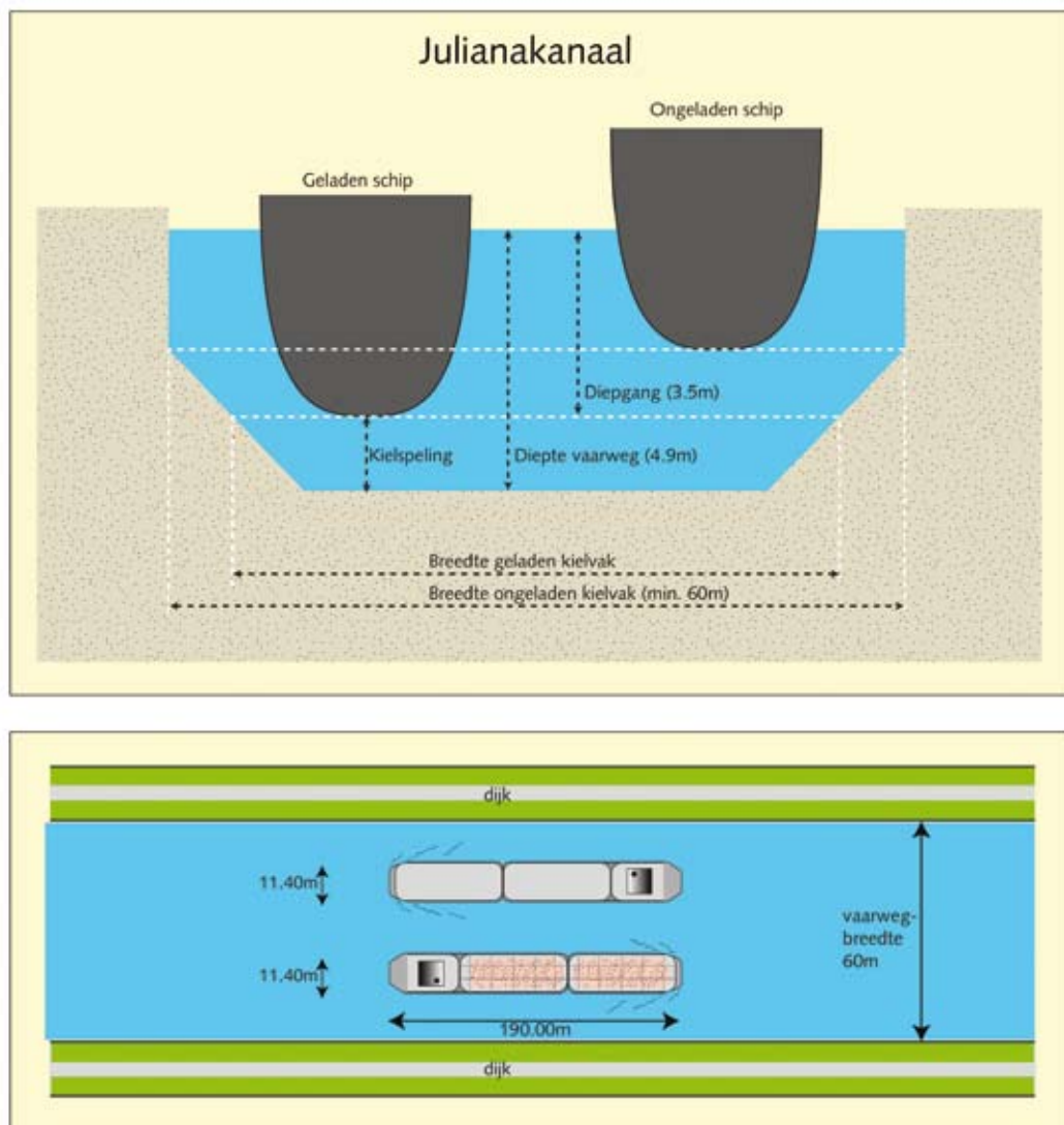
Figuur 2.5. Uitleg termen kielsingeling, diepgang, geladen en ongeladen kielvak, diepte van de vaarweg, vaarwegbreedte en tweebaksduwvaart behorend bij Vb-klasse vaarweg met een diepgang van 3,5 m.
