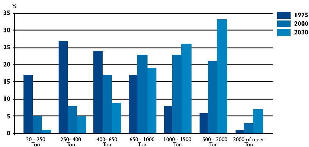
Figuur 2.1. Samenstelling/groei Nederlandse actieve binnenvloot in percentages 2
