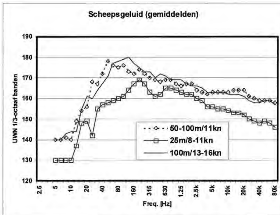
Figuur 24: de gemiddelde bronniveaus ( L_{eq} ) van diverse schepen, gemeten volgens militaire standaards, in 1/3-octaf bandbreedte en in dB re 1 \mu Pa^2 m^2 .
