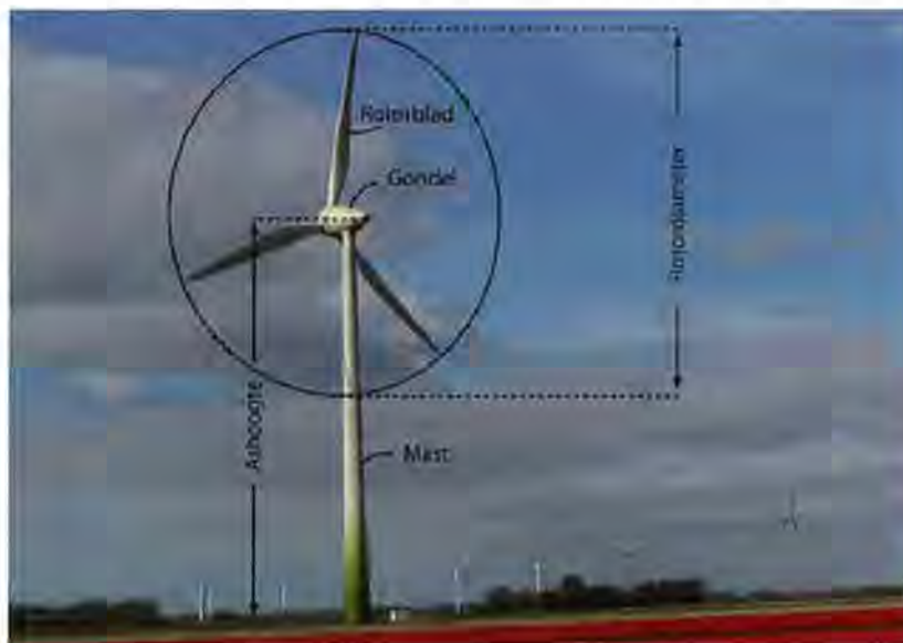
Figuur 3: opbouw van een windturbine
