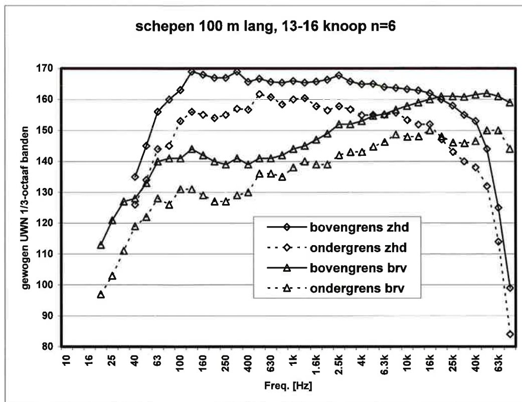
Figuur 26: spreidingsgebied van het uitgestraald geluid van 6 koopvaardijsschepen met een lengte van ca. 100 m en een vaarsnelheid tussen 13 – 16 knoop. Voor zeehond en Bruinvvis gewogen bronniveau in 1/3-octaf banden en in dB re 1 \mu\text{Pa}^2 \text{m}^2 .
