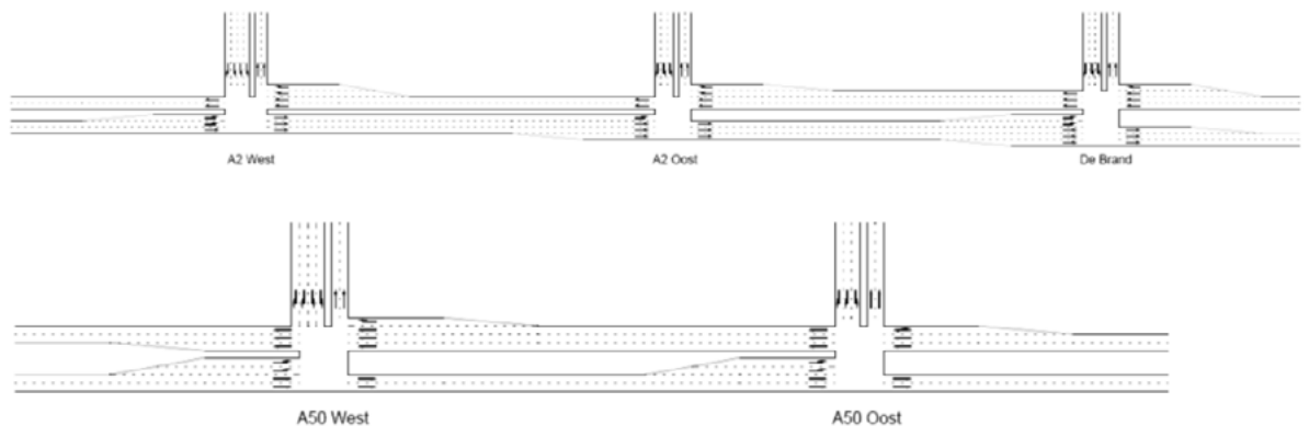
Afbeelding 3.12: Globaal rijstrokschema alternatief B
