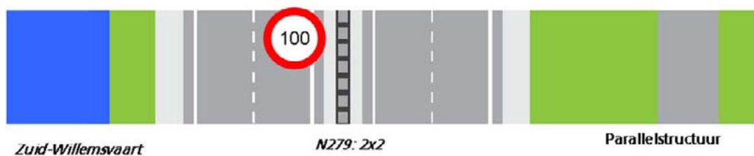
Afbeelding 3.14: Globaal dwarsprofiel alternatief D
