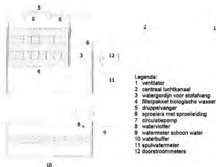
Figuur 26: Schematische weergave van de BWL 2009.12 luchtwasser
