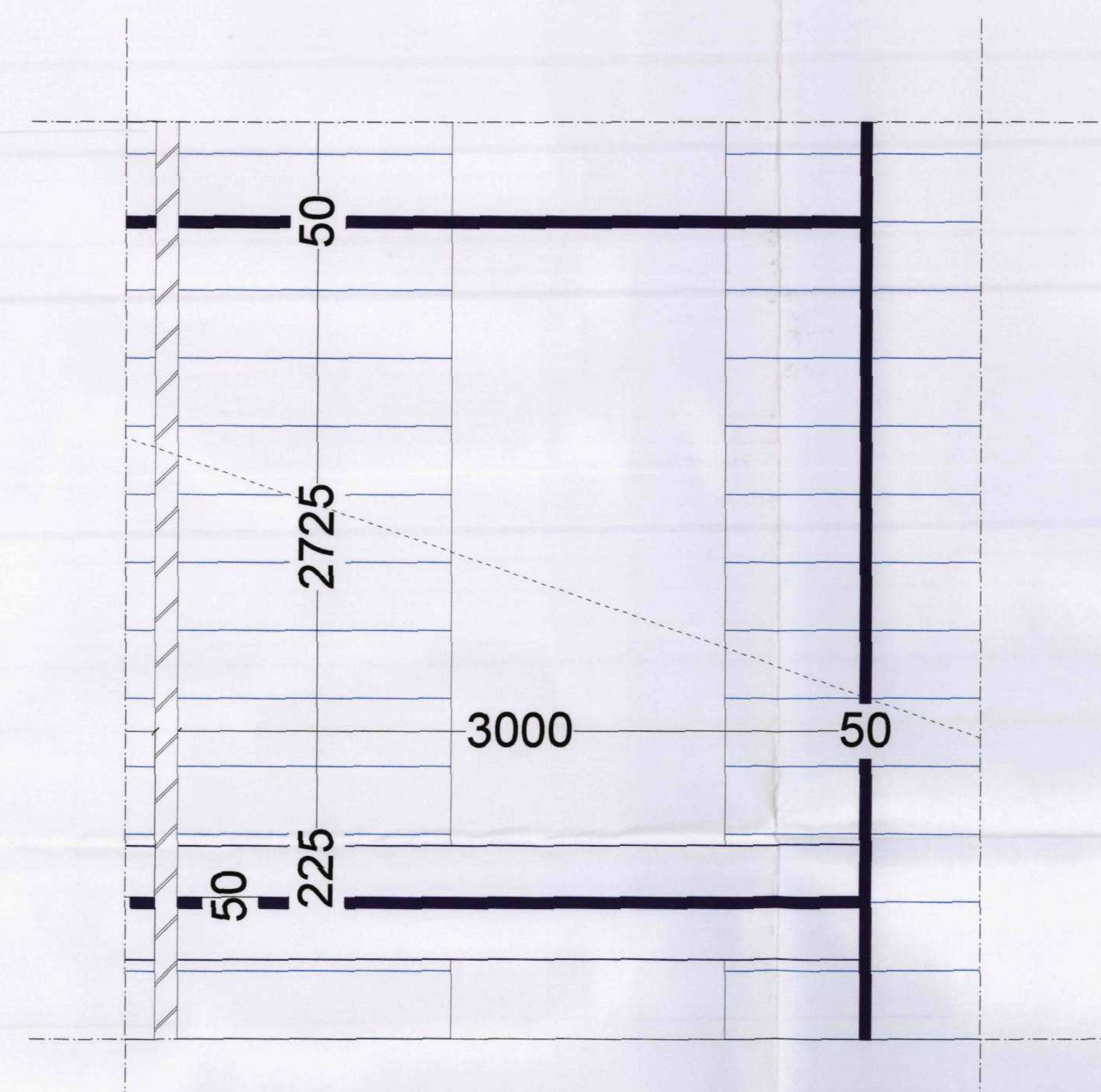
detail 2 (schaal 1:20)
