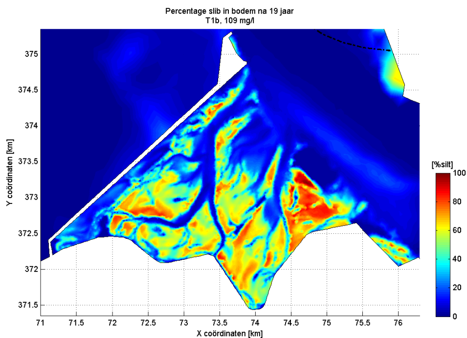
Figuur 3.36: Percentage slib in de toplaag van de bodem aan het eind van de modelberekening voor scenario T1b.
