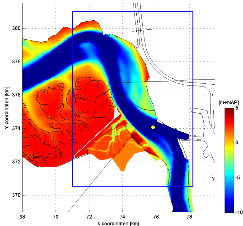
Figuur 2.8: Modelbodem ter plaatse van de Hedwig- en Prosperpolder in de T1 situatie. Het blauwe kader toont het morfologisch actieve gebied. De gele punt geeft de slibmeetlocatie bij Schaar van Ouden Doel aan.
