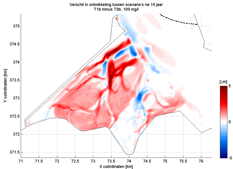
Figuur 3.17: Vershil in bodemontwikkeling tussen scenario T1b en T0b. In de rode gebieden treedt in T1a meer sedimentatie/minder erosie op dan in T0b; in de blauwe gebieden treedt in T1a minder sedimentatie/meer erosie op dan in T0b.
