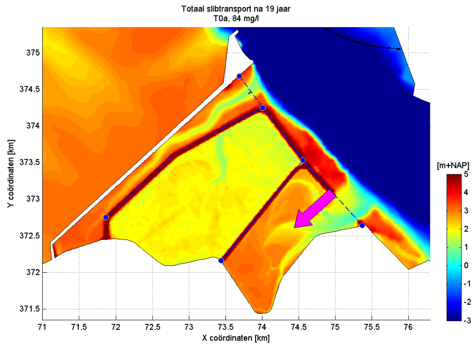
Figuur 3.23: Cumulatief slijbtransport door enkele dwarsdoorsneden in de Hedwig- en Prosperpolder aan het eind van de modelberekening voor scenario T0a.
