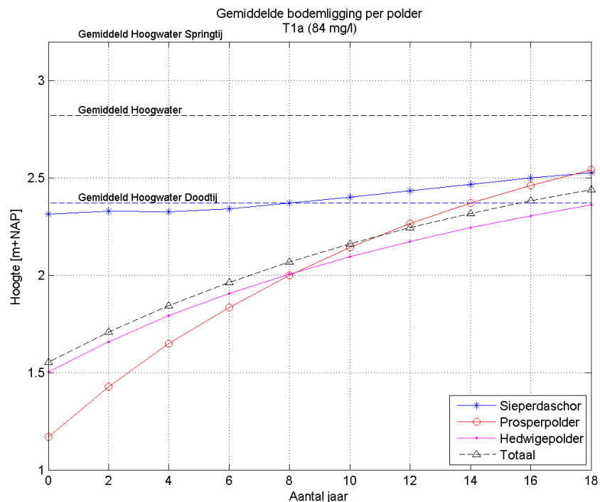
Figuur 3.14: Gemiddelde hoogte in de afzonderlijke polders voor scenario T1a. Geulen zijn in het gemiddelde meegenomen, dijken niet. De gemiddelde hoogwaterstand bij gemiddeld tij, springtij en doottij zijn eveneens gepresenteerd.
