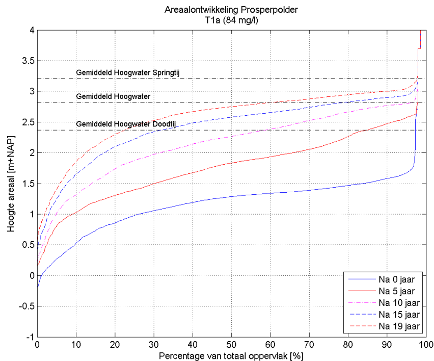
Figuur 3.42: Hypsometrische curve van de Prosperpolder voor verschillende momenten in scenario T1a. De gemiddelde hoog- en laagwaterstand bij gemiddeld tij, springtij en doottij zijn eveneens gepresenteerd .
