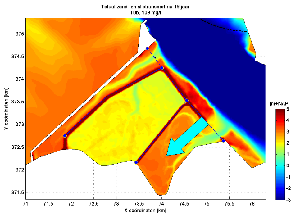
Figuur 3.26: Cumulatief zand- en slibtransport door enkele dwarsdoorsneden in de Hedwig- en Prosperpolder aan het eind van de modelberekening voor scenario T0b.
