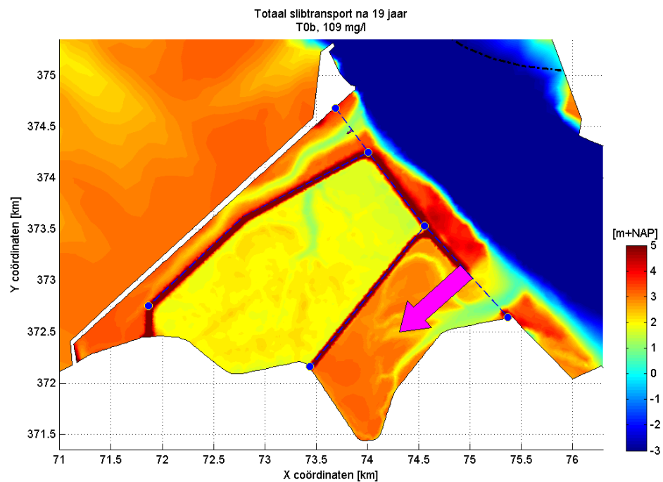
Figuur 3.24: Cumulatief slijbtransport door enkele dwarsdoorsneden in de Hedwig- en Prosperpolder aan het eind van de modelberekening voor scenario T0b.
