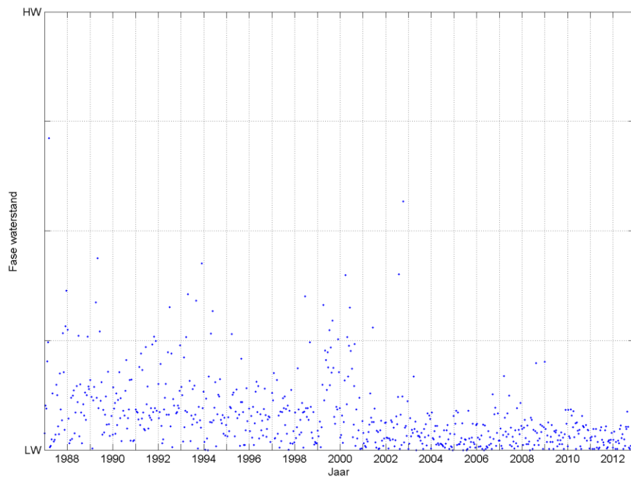
Figuur 2.10: Moment van monsternamen van de slibmonsters bij Schaar van Ouden Doel ten opzichte van waterstand bij Bath. Weergegeven wordt hoe dicht het monsternamemoment bij het dichtstbijzijnde hoogwater- en laagwatertijdstip ligt. Het faseverschil tussen Bath en Schaar van Ouden Doel bedraagt enkele minuten.
