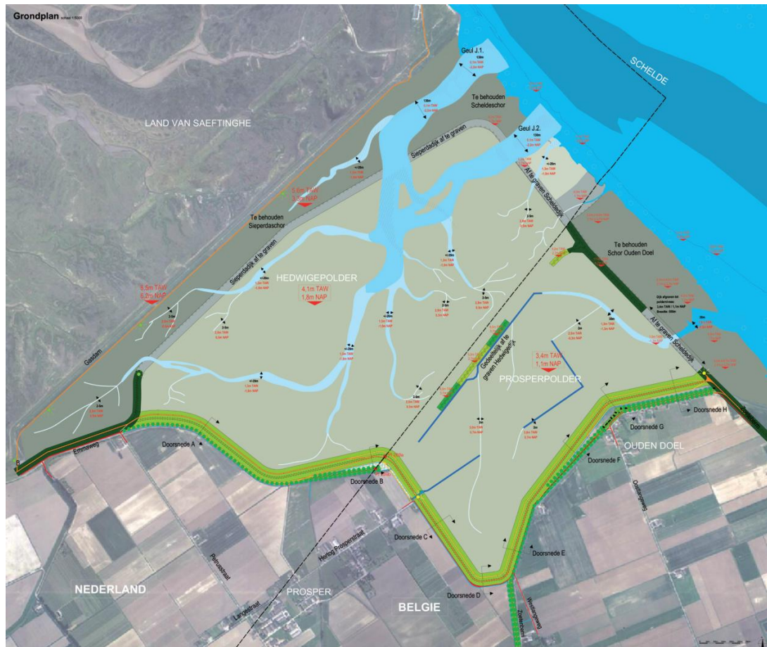
Figuur 1.1: Inrichtingsplan voor de Hedwigepolder als gepresenteerd door de Provincie Zeeland op 25 juni 2013.
