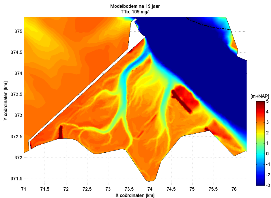
Figuur 3.10: Bodem aan het eind van de berekening voor scenario T1b.
