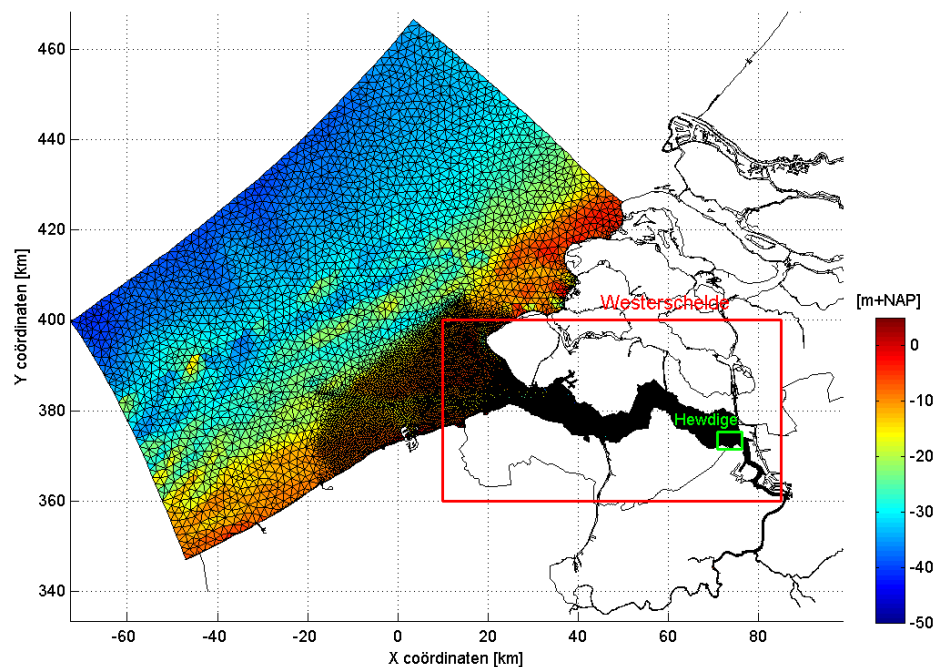
Figuur 2.1: Rekenrooster van FINEL2D Westerschelde model. In Figuur 2.2 wordt het deel van het rekenrooster in het rode kader weergegeven; in Figuur 2.3 het deel in het groene kader.
