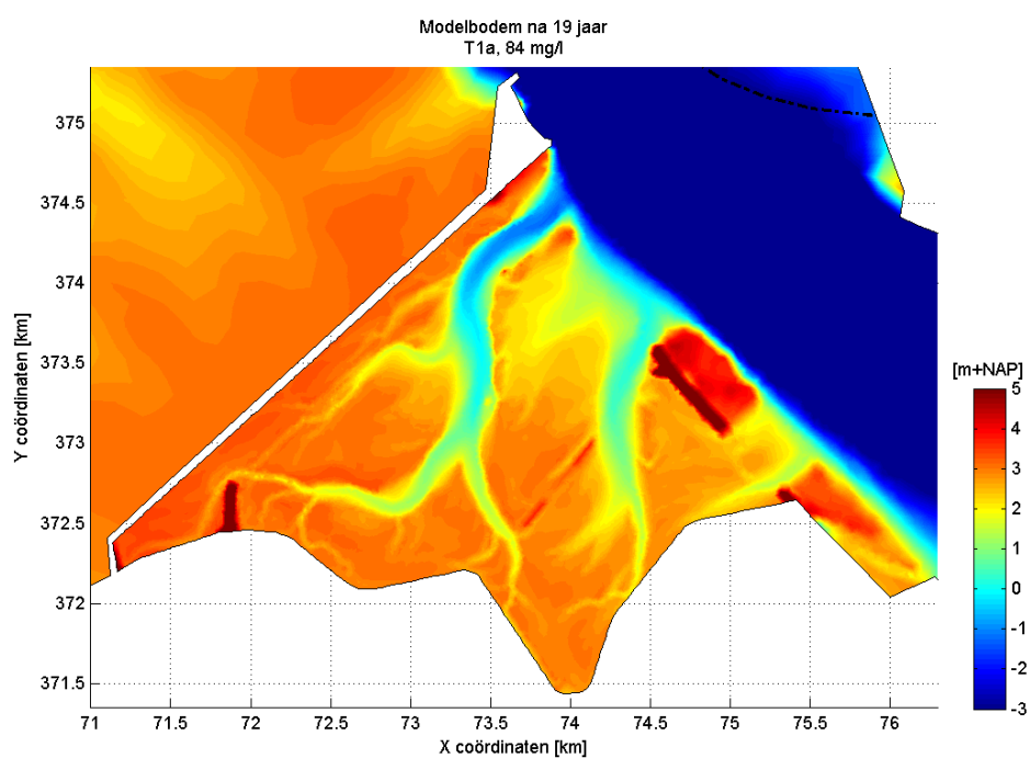
Figuur 3.9: Bodem aan het eind van de berekening voor scenario T1a.
