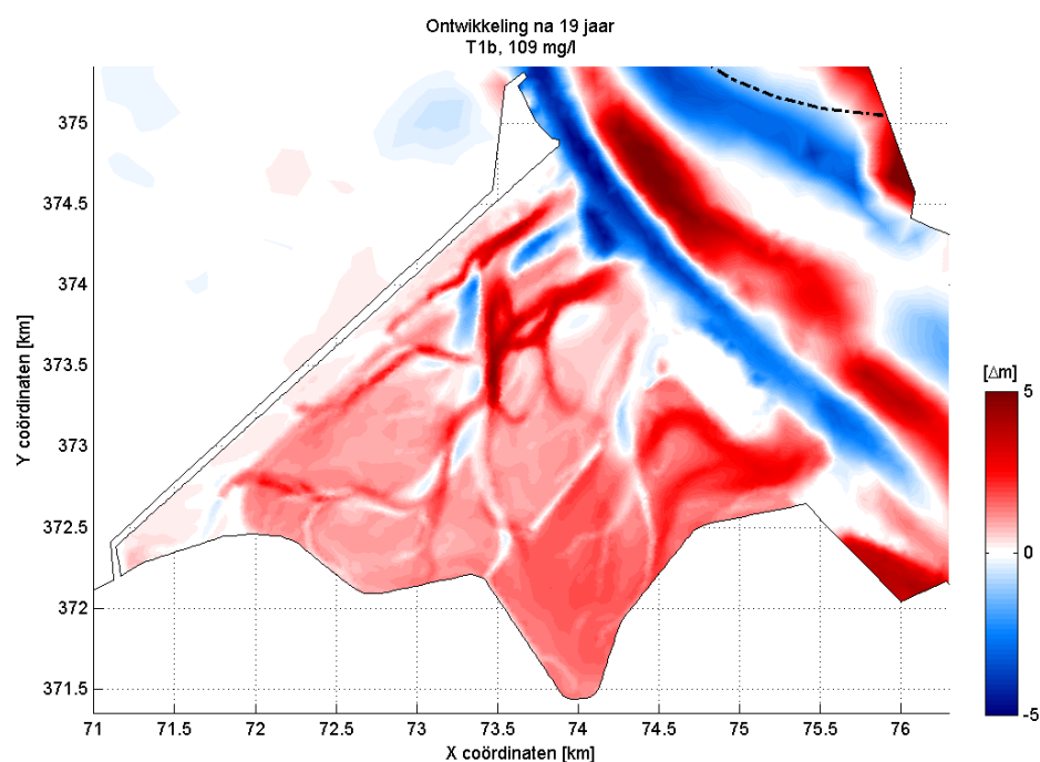
Figuur 3.12: Bodemontwikkeling na 19 jaar voor scenario T1b. In de rode gebieden treedt sedimentatie op; in de blauwe erosie.
