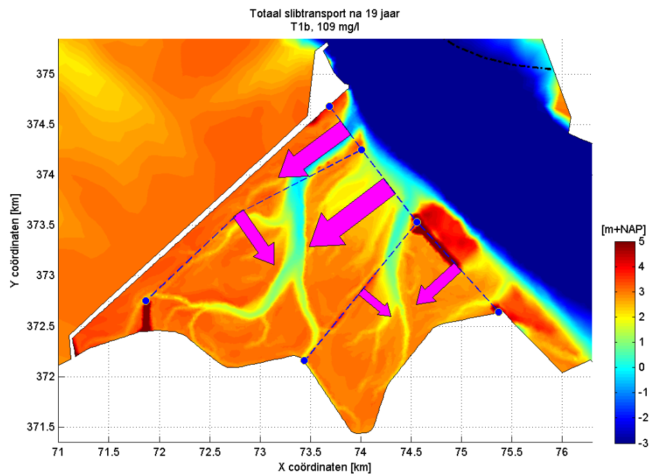
Figuur 3.32: Cumulatief slijbtransport door enkele dwarsdoorsneden in de Hedwig- en Prosperpolder aan het eind van de modelberekening voor scenario T1b.
