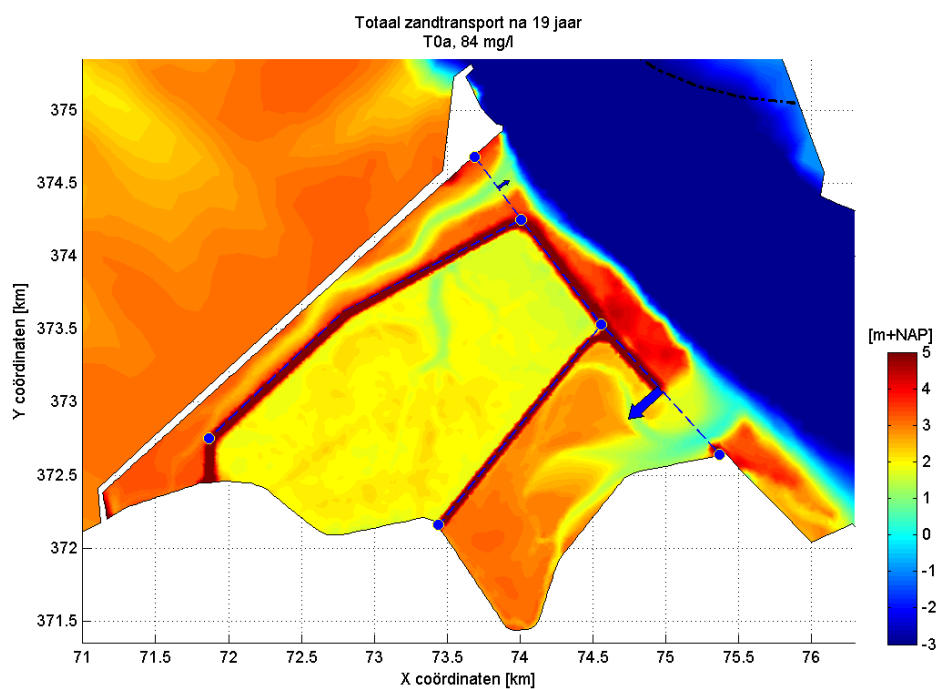
Figuur 3.21: Cumulatief zandtransport door enkele dwarsdoorsneden in de Hedwige- en Prosperpolder aan het eind van de modelberekening voor scenario T0a.
