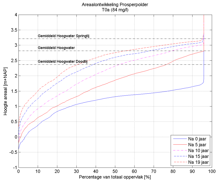
Figuur 3.39: Hypsometrische curve van de Prosperpolder voor verschillende momenten in scenario T0a. De gemiddelde hoog- en laagwaterstand bij gemiddeld tij, springtij en doottij zijn eveneens gepresenteerd.
