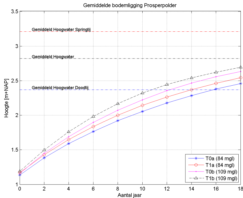
Figuur 3.19: Gemiddelde hoogte in de Prosperpolder voor alle scenario's. Geulen zijn in het gemiddelde meegenomen, dijken niet. De gemiddelde hoogwaterstand bij gemiddeld tij, springtij en doottij zijn eveneens gepresenteerd.
