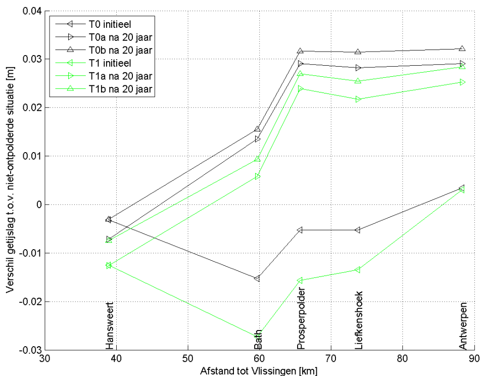
Figuur 3.47: Verschil in getijslag ten opzichte van de huidige situatie zonder ontpolderen voor de scenario's na 0 (initieel) en 20 jaar.
