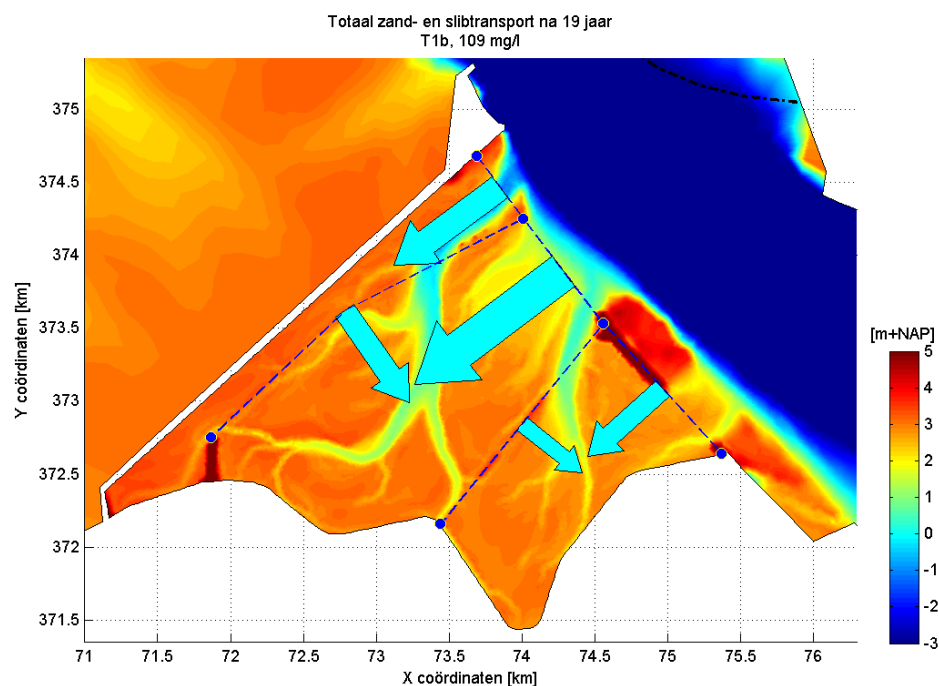
Figuur 3.34: Cumulatief zand- en slibtransport door enkele dwarsdoorsneden in de Hedwig- en Prosperpolder aan het eind van de modelberekening voor scenario T1b.
