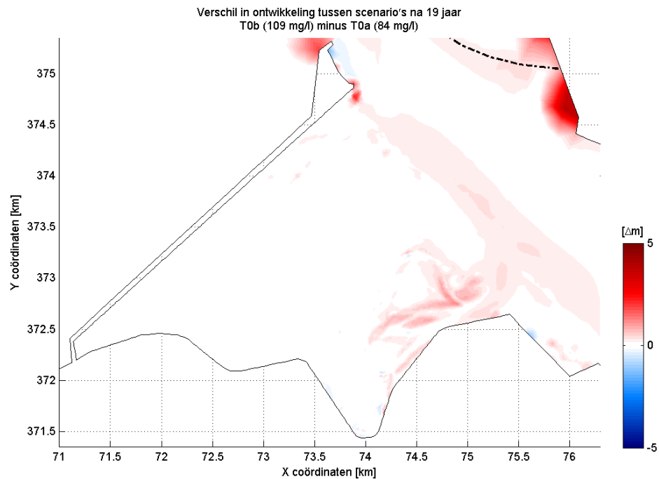
Figuur 3.5: Vershil in bodemontwikkeling tussen beide referentiescenario's na 19 jaar. In de rode gebieden treedt in T0b meer sedimentatie/minder erosie op dan in T0a; in de blauwe gebieden treedt minder sedimentatie/meer erosie op in T0b dan in T0a.
