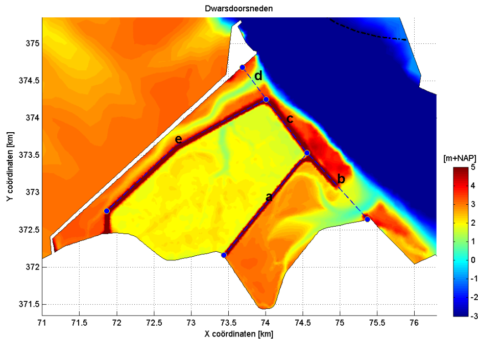
Figuur 3.20: Dwarsdoorsneden gebruikt voor de bepaling van sedimenttransporten in de verschillende polders.
