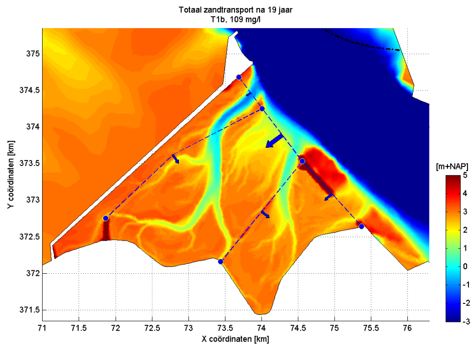
Figuur 3.30: Cumulatief zandtransport door enkele dwarsdoorsneden in de Hedwig- en Prosperpolder aan het eind van de modelberekening voor scenario T1b.
