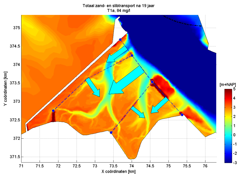
Figuur 3.33: Cumulatief zand- en slibtransport door enkele dwarsdoorsneden in de Hedwig- en Prosperpolder aan het eind van de modelberekening voor scenario T1a.
