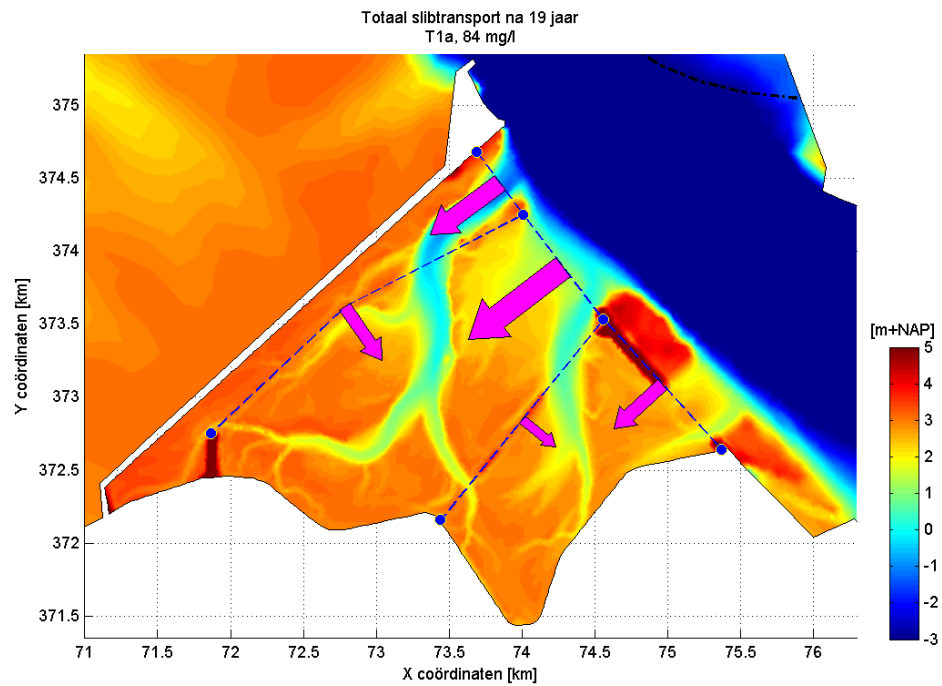
Figuur 3.31: Cumulatief slijbtransport door enkele dwarsdoorsneden in de Hedwig- en Prosperpolder aan het eind van de modelberekening voor scenario T1a.
