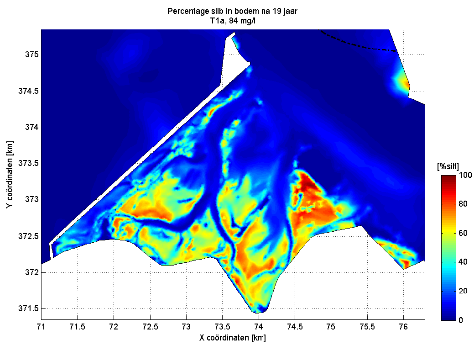
Figuur 3.35: Percentage slib in de toplaag van de bodem aan het eind van de modelberekening voor scenario T1a.
