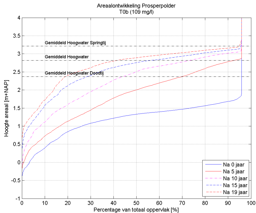
Figuur 3.40: Hypsometrische curve van de Prosperpolder voor verschillende momenten in scenario T0b. De gemiddelde hoog- en laagwaterstand bij gemiddeld tij, springtij en doottij zijn eveneens gepresenteerd.
