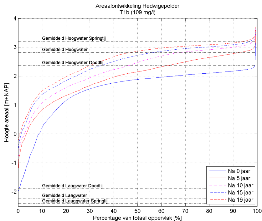
Figuur 3.43: Hypsometrische curve van de Hedwigepolder voor verschillende momenten in scenario T1b. De gemiddelde hoog- en laagwaterstand bij gemiddeld tij, springtij en doottij zijn eveneens gepresenteerd.
