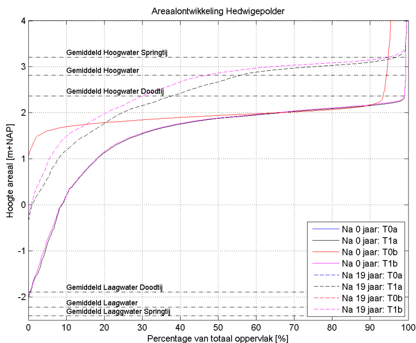
Figuur 3.45: Hypsometrische curve van de Hedwigepolder aan het begin en eind van de berekening van de verschillende scenario's. De gemiddelde hoog- en laagwaterstand bij gemiddeld tij, springtij en doodtij zijn eveneens gepresenteerd.
