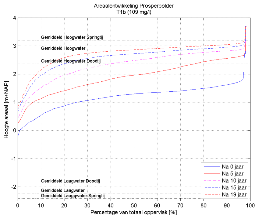
Figuur 3.44: Hypsometrische curve van de Prosperpolder voor verschillende momenten in scenario T1b. De gemiddelde hoog- en laagwaterstand bij gemiddeld tij, springtij en doottij zijn eveneens gepresenteerd.
