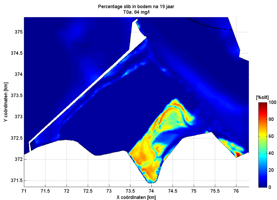
Figuur 3.27: Percentage silt in de toplaag van de bodem aan het eind van de modelberekening voor scenario T0a.
