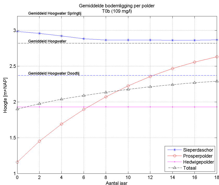
Figuur 3.7: Gemiddelde hoogte in de afzonderlijke polders voor scenario T0b. Geulen zijn in het gemiddelde meegenomen, dijken niet. De gemiddelde hoogwaterstand bij gemiddeld tij, springtij en doortij zijn eveneens gepresenteerd.
