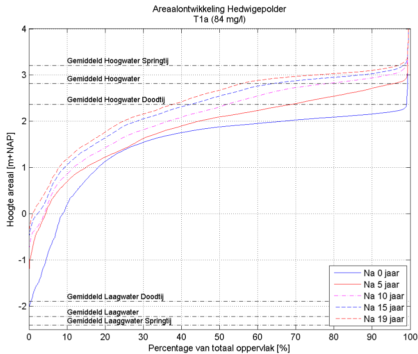
Figuur 3.41: Hypsometrische curve van de Hedwigepolder voor verschillende momenten in scenario T1a. De gemiddelde hoog- en laagwaterstand bij gemiddeld tij, springtij en doottij zijn eveneens gepresenteerd .
