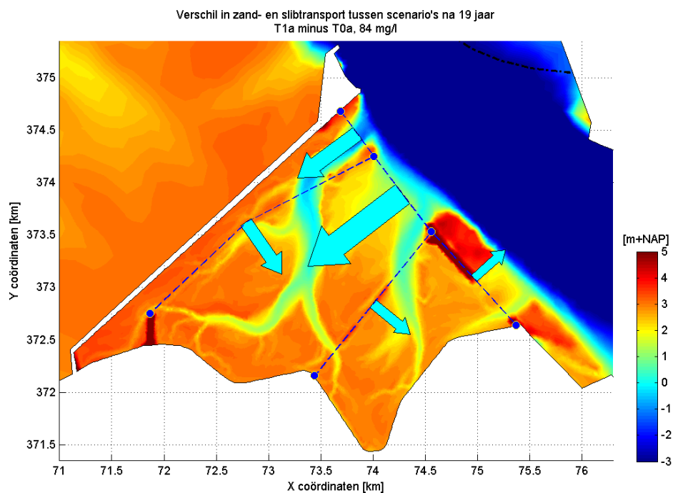
Figuur 3.37: Verschil in cumulatief zand- en slibtransport tussen scenario T1a en T0a door enkele dwarsdoorsneden in de Hedwige- en Prosperpolder aan het eind van de modelberekening.
