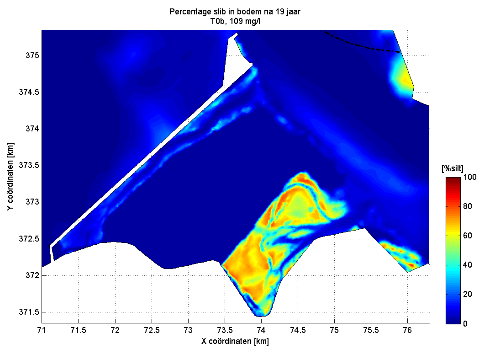
Figuur 3.28: Percentage silt in de toplaag van de bodem aan het eind van de modelberekening voor scenario T0b.
