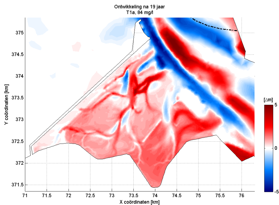
Figuur 3.11: Bodemontwikkeling na 19 jaar voor scenario T1a. In de rode gebieden treedt sedimentatie op; in de blauwe erosie.
