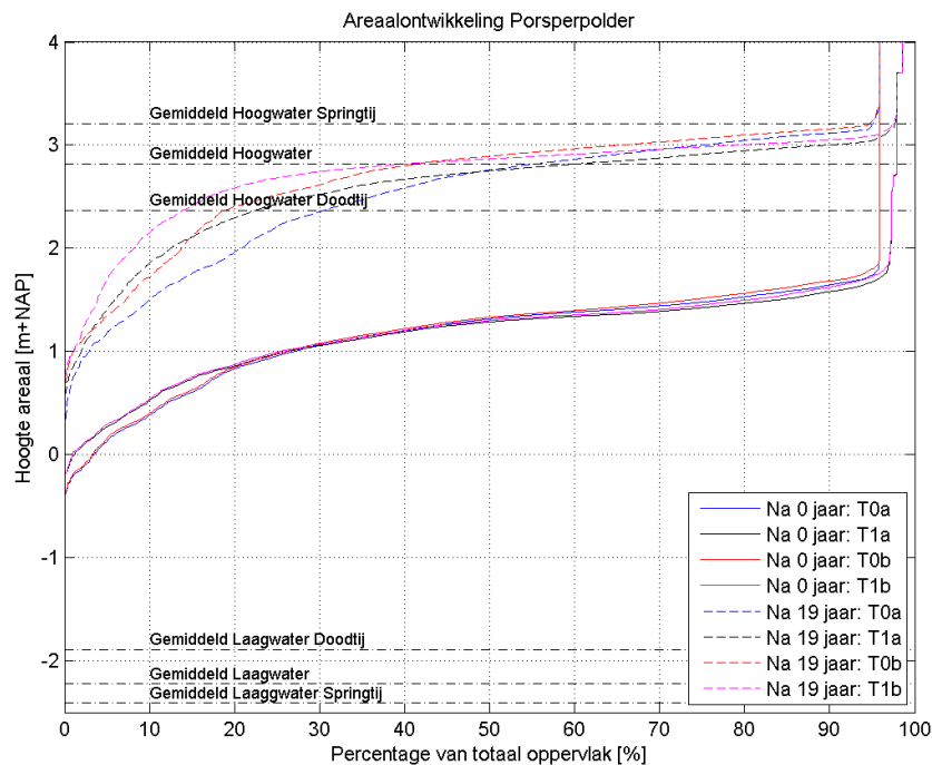
Figuur 3.46: Hypsometrische curve van de Prosperpolder aan het begin en eind van de berekening van de verschillende scenario's. De gemiddelde hoog- en laagwaterstand bij gemiddeld tij, springtij en doottij zijn eveneens gepresenteerd.
