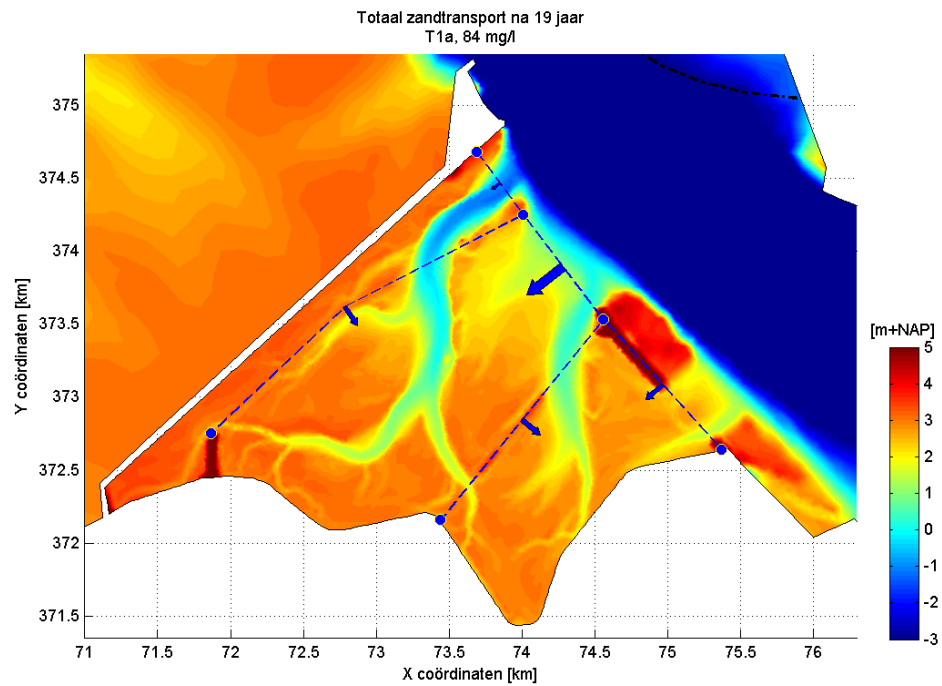
Figuur 3.29: Cumulatief zandtransport door enkele dwarsdoorsneden in de Hedwig- en Prosperpolder aan het eind van de modelberekening voor scenario T1a.
