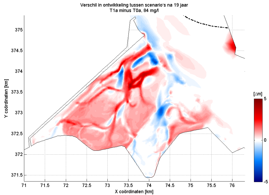
Figuur 3.16: Vershil in bodemontwikkeling tussen scenario T1a en T0a. In de rode gebieden treedt in T1a meer sedimentatie/minder erosie op dan in T0a; in de blauwe gebieden treedt in T1a minder sedimentatie/meer erosie op dan in T0a.
