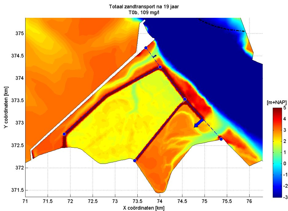
Figuur 3.22: Cumulatief zandtransport door enkele dwarsdoorsneden in de Hedwige- en Prosperpolder aan het eind van de modelberekening voor scenario T0b.
