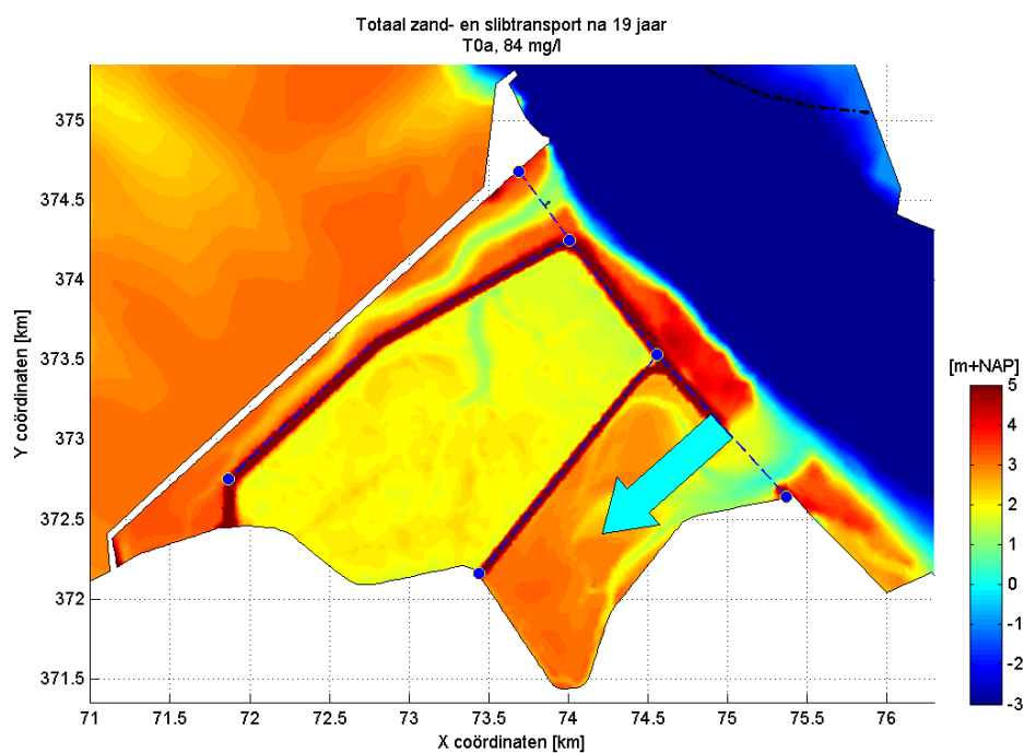
Figuur 3.25: Cumulatief zand- en slibtransport door enkele dwarsdoorsneden in de Hedwig- en Prosperpolder aan het eind van de modelberekening voor scenario T0a.
