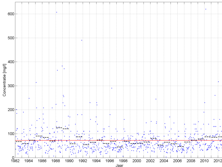
Figuur 2.9: Slibconcentratie bij Schaar van Ouden Doel (Rijkswaterstaat). De metingen zijn vrijwel allemaal rond laagwater genomen. De rode lijn geeft de gemiddelde concentratie over de gehele periode. De zwart gestreepte lijnen geven de gemiddelde concentratie in elk afzonderlijk jaar.
