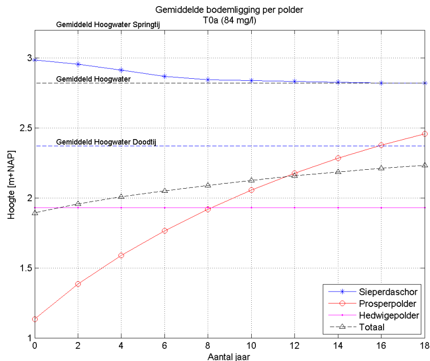
Figuur 3.6: Gemiddelde hoogte in de afzonderlijke polders voor scenario T0a. Geulen zijn in het gemiddelde meegenomen, dijken niet. De gemiddelde hoogwaterstand bij gemiddeld tij, springtij en doottij zijn eveneens gepresenteerd.
