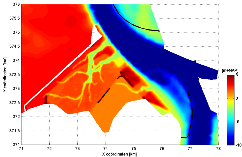
Figuur 2.7: Initiële modelbodem ter plaatse van de Hedwigepolder en Prosperpolder in de T1 situatie. De zwarte lijnen tonen de locatie van de leidammen en de delen van de Hedwigedijk die als overlaat in de berekening zijn meegenomen.
