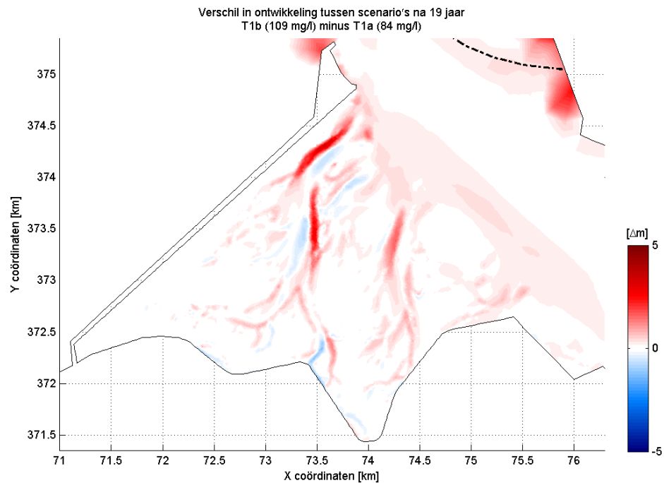
Figuur 3.13: Verschil in bodemontwikkeling tussen beide ontpolderingsscenario's na 19 jaar. In de rode gebieden treedt in T1b meer sedimentatie/minder erosie op dan in T1a; in de blauwe gebieden treedt minder sedimentatie/meer erosie op in T1b dan in T1a.
