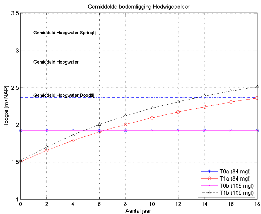
Figuur 3.18: Gemiddelde hoogte in de Hedwigepolder voor alle scenario's. Geulen zijn in het gemiddelde meegenomen, dijken niet. De gemiddelde hoogwaterstand bij gemiddeld tij, springtij en doottij zijn eveneens gepresenteerd.
