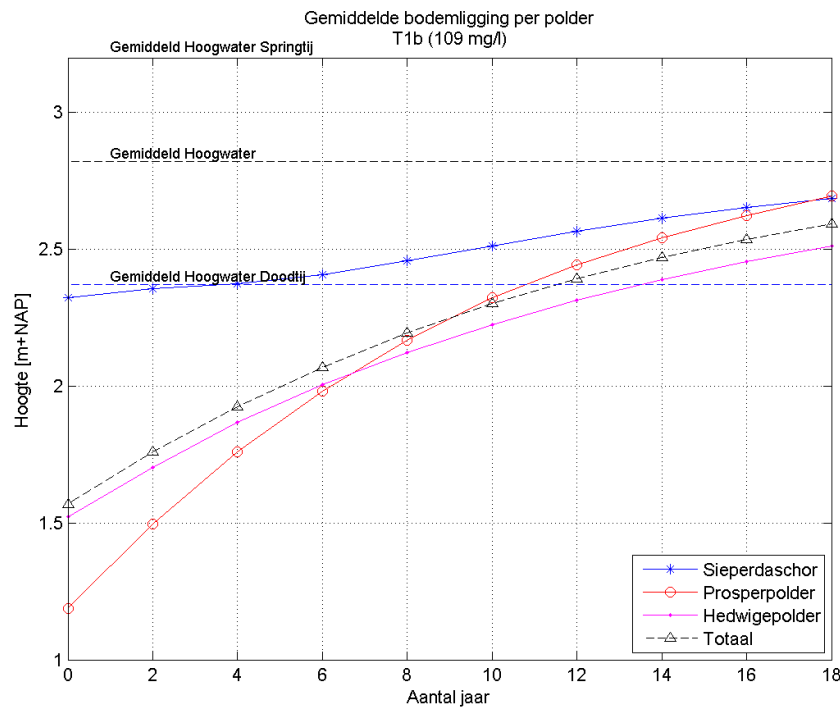
Figuur 3.15: Gemiddelde hoogte in de afzonderlijke polders voor scenario T1b. Geulen zijn in het gemiddelde meegenomen, dijken niet. De gemiddelde hoogwaterstand bij gemiddeld tij, springtij en doottij zijn eveneens gepresenteerd.
