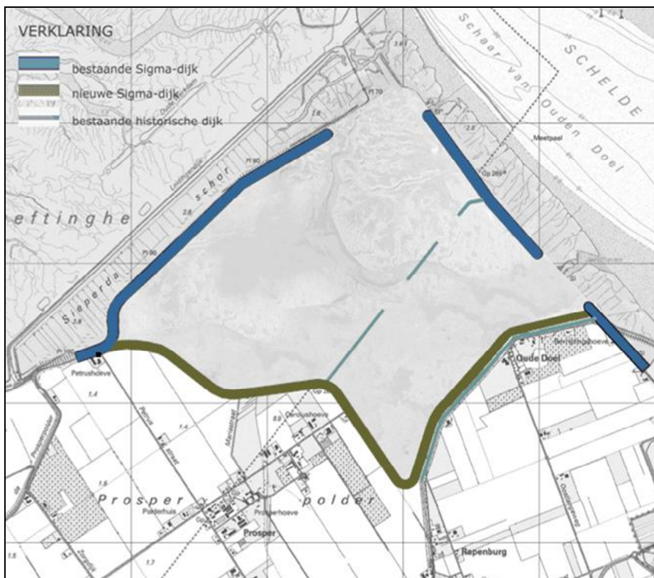
Figuur 2.2: Basisalternatief 1: realisatie van bressen door het afgraven van dijkdelen tot op polderniveau.
