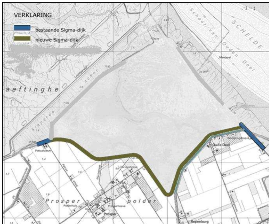
Figuur 2.4: Basisalternatief 3: afgraven van de Scheldedijk, Sieperdadijk en Hedwigidijk tot op polderniveau.
