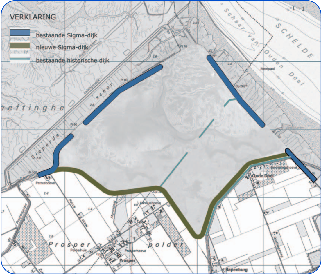
> Figuur 4-3: Basisalternatief 2, variant met bres achteraan het Sieperdaschor
