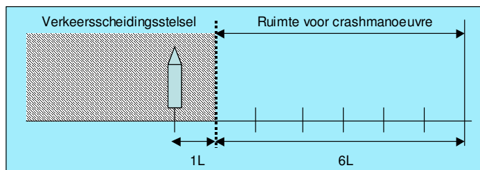
Figuur 3: Benodigde ruimte voor een uitwijk(crash)manoeuvre voor schepen die aan stuurboordzijde van de verkeersbaan in een verkeersscheidingssysteem varen.
