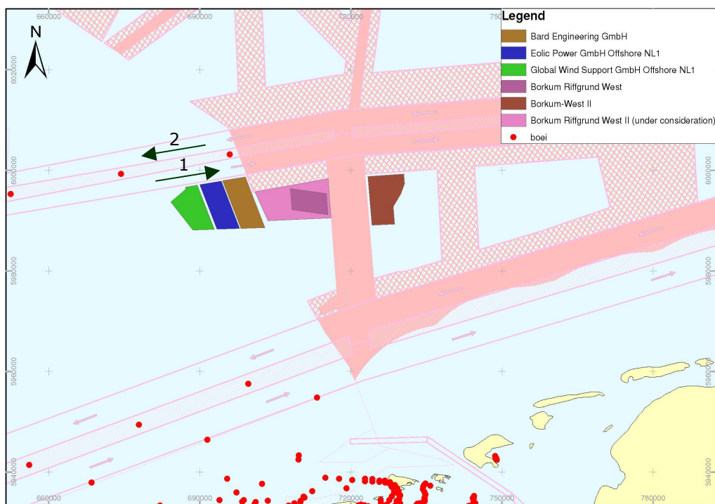
Figuur 1: ligging van windpark BARD Offshore NL1 (bruin) ten opzichte van verkeersstromen 1 en 2 (zwarte pijlen). De roze pijlen geven de verkeersstromen aan in de verkeersscheidingstelsels. [bron: GIS bestanden RWS Noordzee en Bundesamt für Seeschifffahrt und Hydrographie (Duitsland)]
