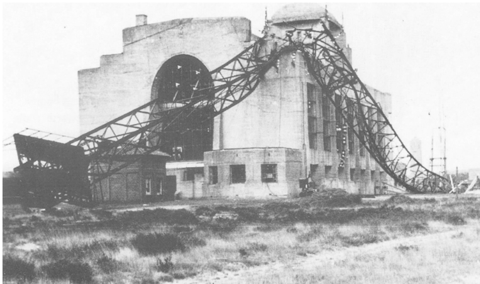
Neergestorte zendmast op gebouw A als gevolg van opblazen van de tuien door de duitsse bezetter aan het eind van de tweede wereldoorlog
