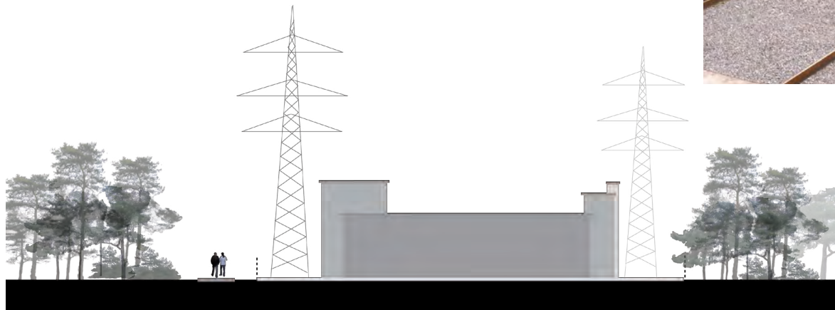
Principeprofiel 50KV-station als afgebakende open ruimte in het verder besloten bosgebied
