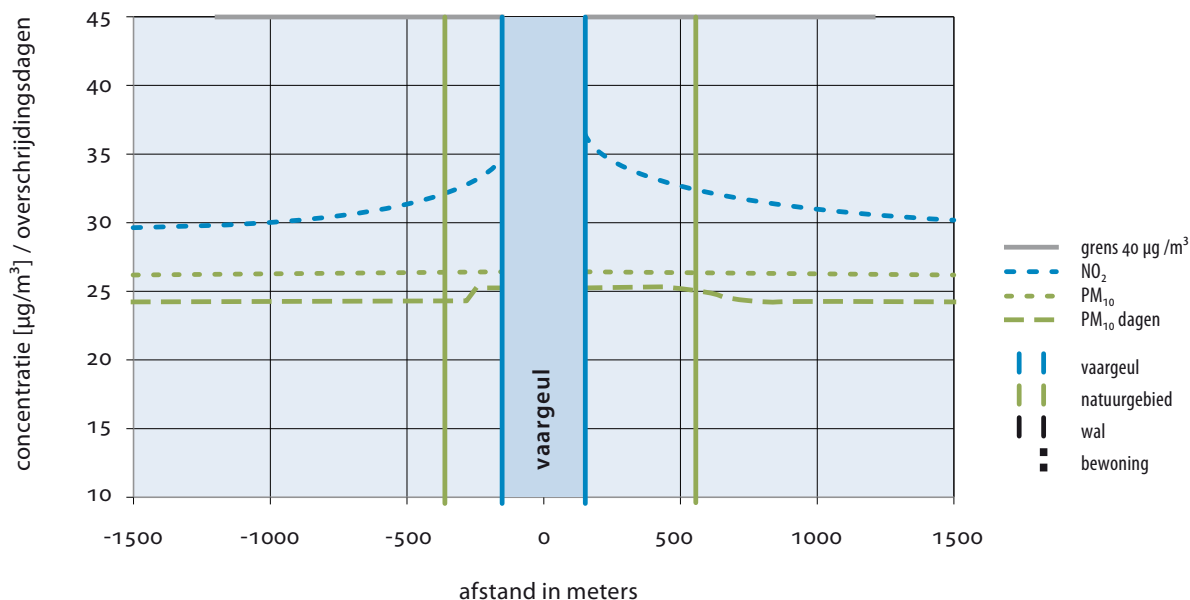
figuur 10-4 \text{NO}_2 en \text{PM}_{10} concentratie en overschrijdingsdagen \text{PM}_{10} , ter hoogte van dwarsprofiel 5, op Nederlands grondgebied
