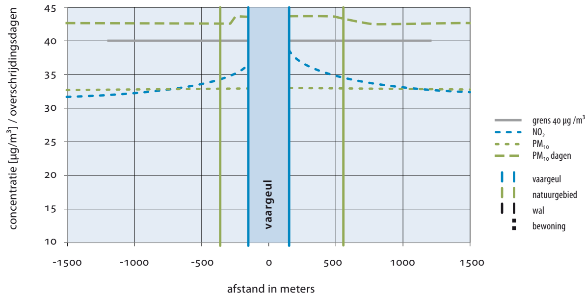
figuur 10-5 NO 2 en PM 10 concentratie en overschrijdingsdagen PM 10 , ter hoogte van dwarsprofiel 5, op Belgisch grondgebied
