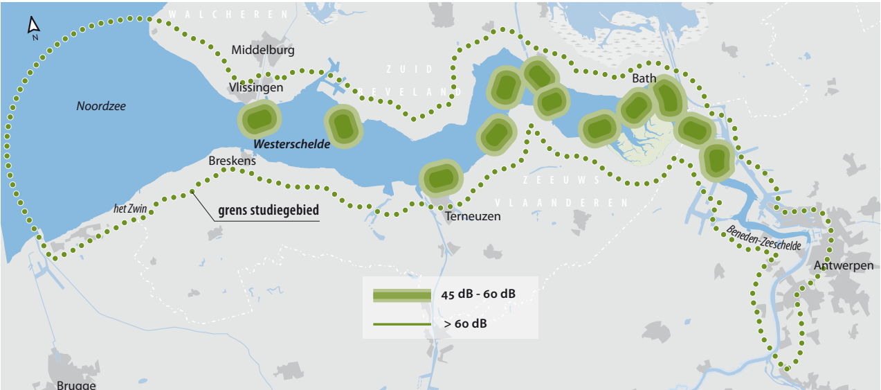
figuur 10-10 Geluidswaarden bij baggeren met schepen die kleppen
