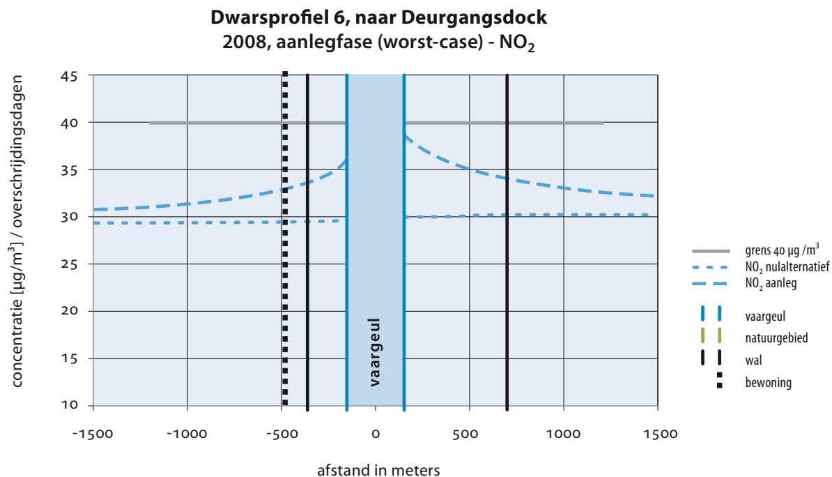
figuur 10-9 NO 2 concentratie bij aanlegfase (2008) ter hoogte van dwarsprofiel 6 op Belgisch grondgebied
