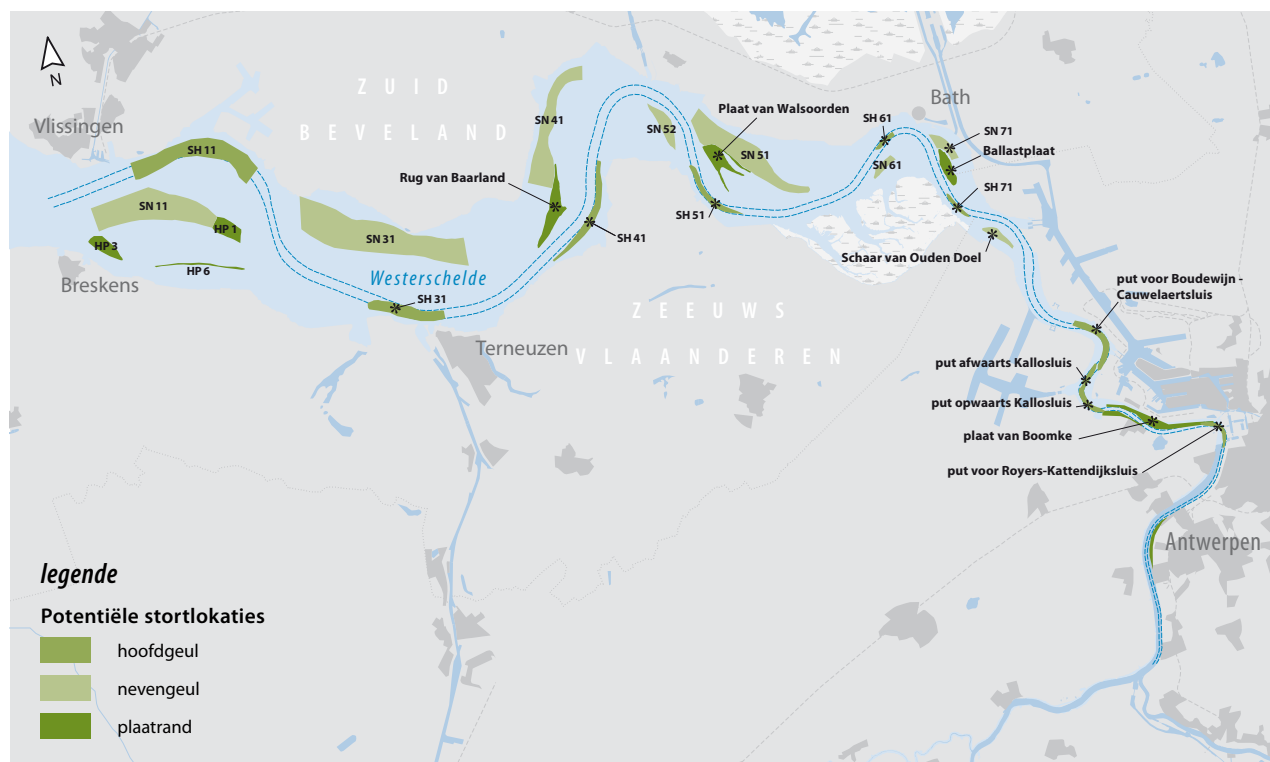
figuur B.10-1 Mogelijke stortzones aanleg- en onderhoudsbaggerspecie
