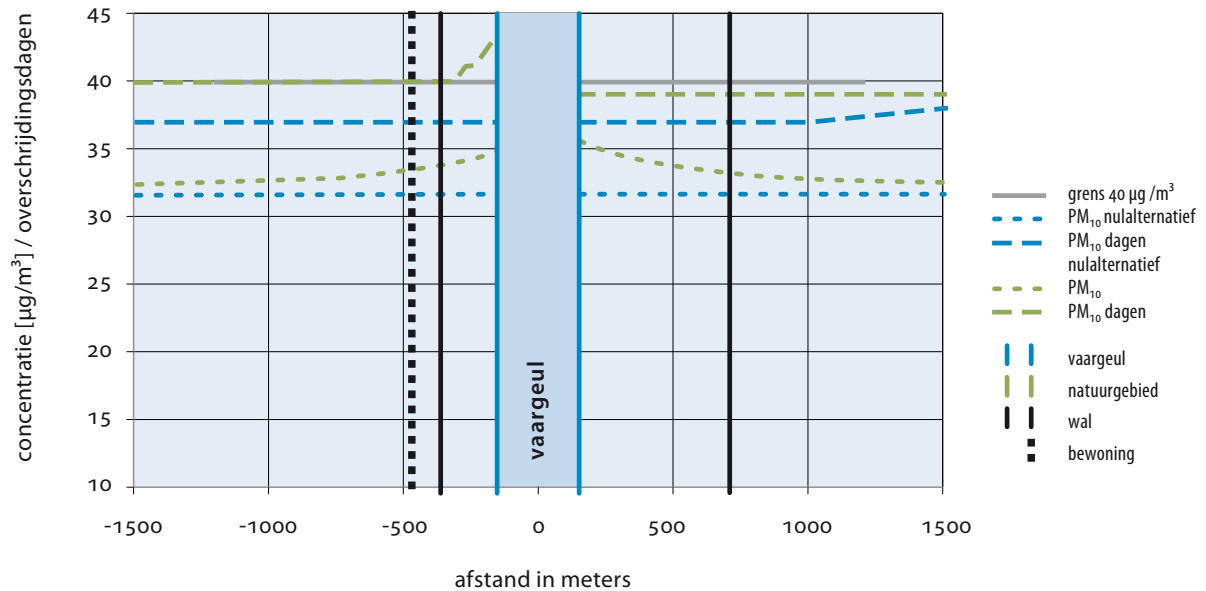
figuur 10-7 PM 10 concentratie bij aanlegfase (2008) ter hoogte van dwarsprofiel 6, op Belgisch grondgebied
