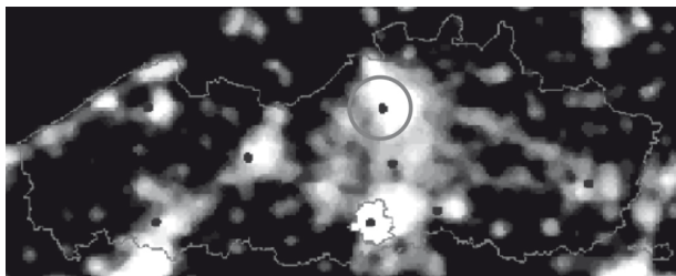
figuur 10-17 Lichtvervuiling Vlaanderen waargenomen vanuit de ruimte in 1994-1995 (Van Steertegem, 2006)
