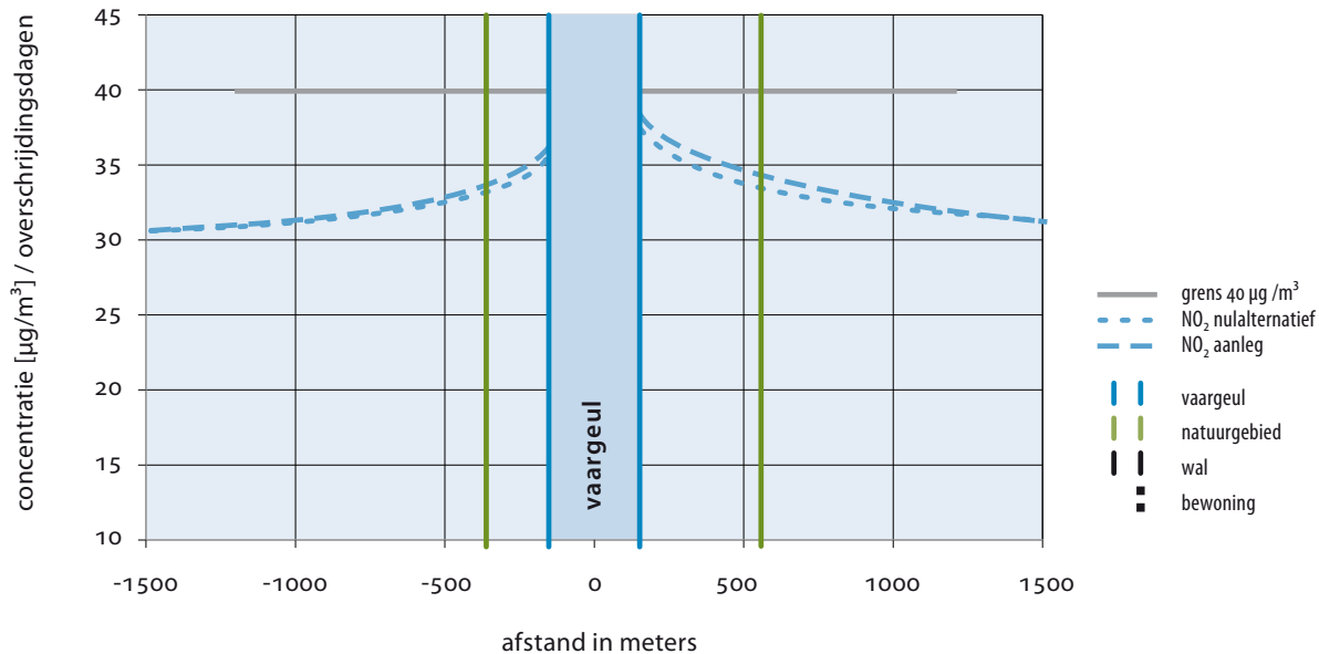
figuur 10-8 NO 2 concentratie bij aanlegfase (2008) ter hoogte van dwarsprofiel 5, op Belgisch grondgebied
