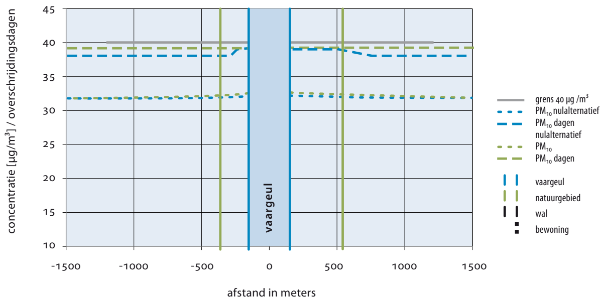
figuur 10-6 PM 10 concentratie bij aanlegfase (2008) ter hoogte van dwarsprofiel 5, op Belgisch grondgebied
