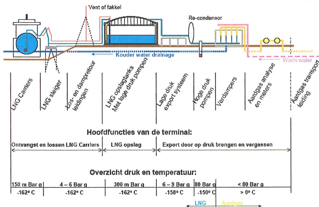
Figuur 2.4: Hoofddcomponenten en -functies van de LNG-terminal
