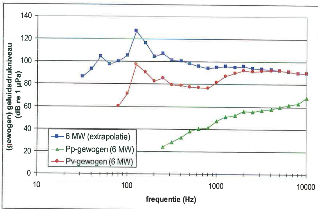
Figuur 16: op metingen in het windpark Paludans Flak gebaseerde ongewogen en audiogram gewogen geluidsspectra op 100 m van de windturbine; frequentie in tertsbanden; Pp = Bruinvis ( Phocoena phocoena ); Pv = Gewone zeehond ( Phoca vitulina )
