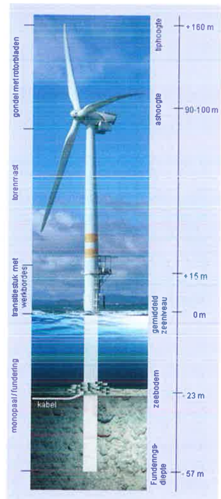
Figuur 3: opbouw van de windturbine (6 MW)
