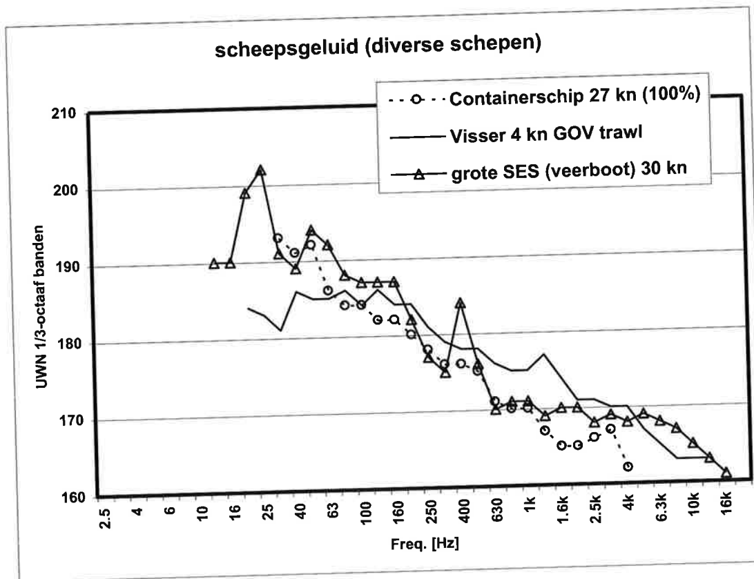
Figuur 25: de gemiddelde bronniveaus ( L_{eq} ) van diverse schepen, gemeten in 1/3-octaf bandbreedte en in dB re 1 \mu\text{Pa}^2 \text{m}^2 .
