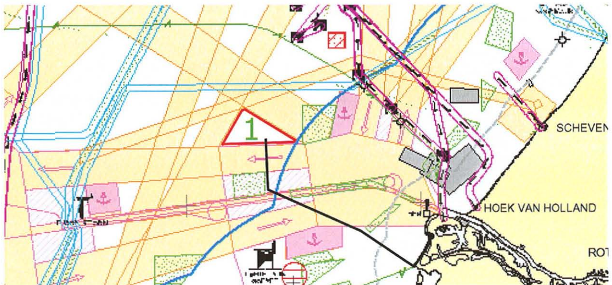
Figuur 1.1 Situering van het project Hoek van Holland 1 met indicatief voorkeustracé aanlandingskabel
