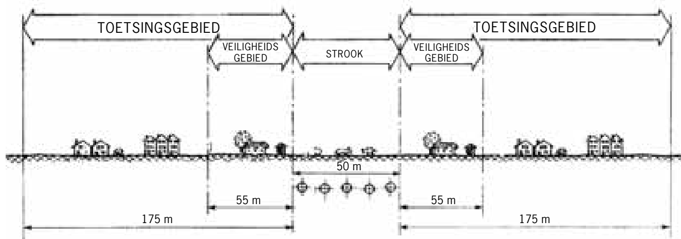
Figuur 6.4 Leidingstroken (incl. bijbehorende zones)
