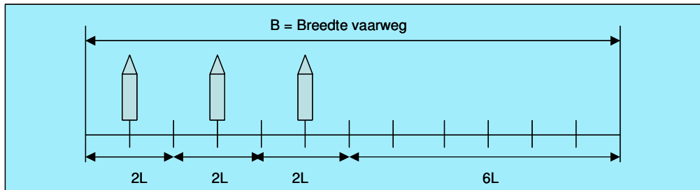
Figuur 3: Minimale breedte van een vaarweg waarin 3 schepen van 400m lengte elkaar kunnen oplopen bedraagt 6 maal ( 3 \times 2 \times 400\text{m} = 2400\text{ m} (= 1,3\text{ NM}) ) om elkaar op voldoende afstand te passeren plus 6 \times 400\text{ m} (= 2400\text{ m} = 1,3\text{ NM}) voor de effectieve draaicirkel in geval van een uitwijk(crash) manoeuvre van 1 schip dus in totaal 2,6 NM. 3
