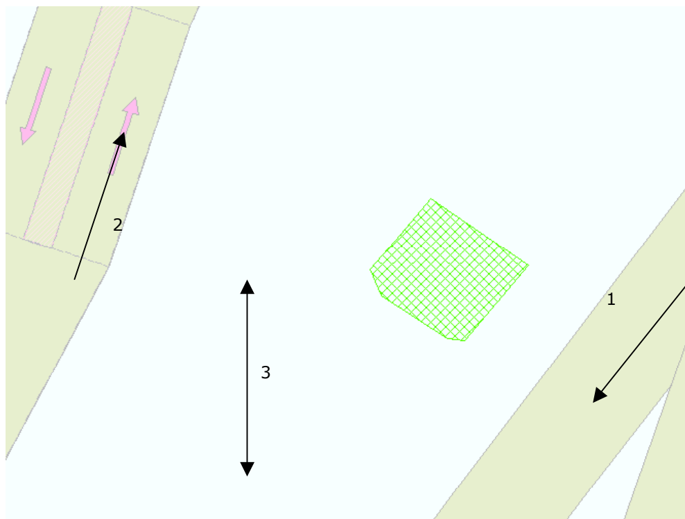
Figuur 1: ligging van windpark Den Helder I (groen) ten opzichte van verkeersstromen 1 t/m 3 (zwarte pijlen). De rose pijlen betreffen een verkeersscheidingsstelsel. [bron: GIS bestanden RWS Noordzee]
