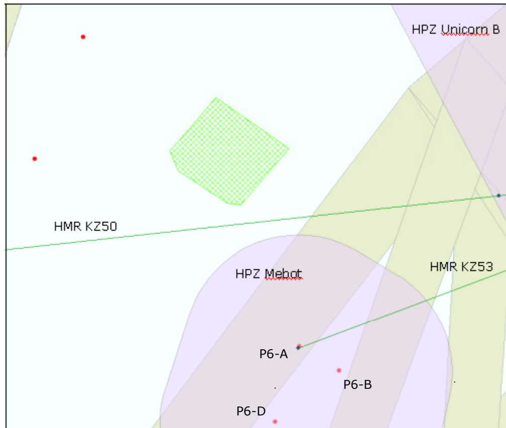
Figuur 4: ligging van Den Helder I (groen gearceerd) t.o.v. platforms met helidek (rood), de HPZ Mebot en HPZ Unicorn B (lichtpaars) en HMR's KZ53 en KZ50 (groene lijnen).
