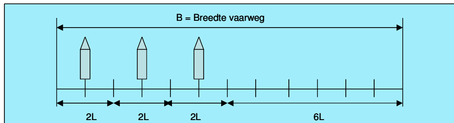
Figuur 3: De minimale breedte van een vaarweg waarin 3 schepen van 400 m lengte elkaar kunnen oplopen bedraagt 6 maal de scheepslengte ( 3 \times 2 \times 400 \text{ m} = 2400 \text{ m} = 1,3 \text{ NM} ) om elkaar te passeren plus 6 scheepslengtes ( = 1,3 \text{ NM} ) voor de effectieve draaicirkel in geval van een uitwijk(crash) manoeuvre van 1 schip en is in totaal dus 2,6 \text{ NM} . 4
