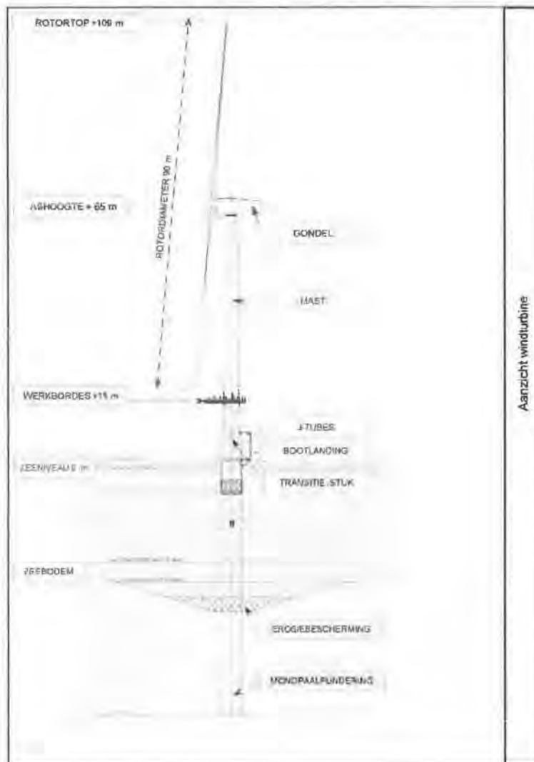
Figuur 3: opbouw van de windturbine (3 MW)
