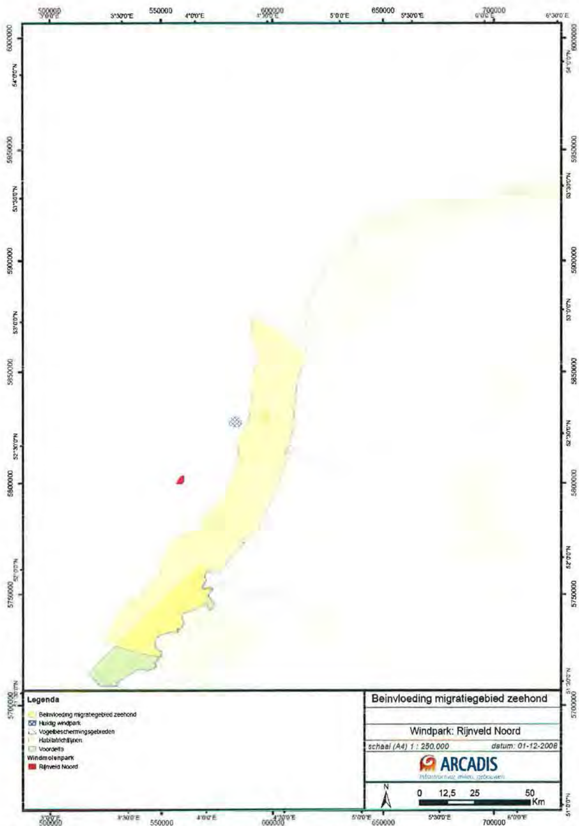
Figuur 20: beïnvloedingsgebied in de kustzone door heiwerkzaamheden in de aanlegfase van windpark Rijnveld Noord
