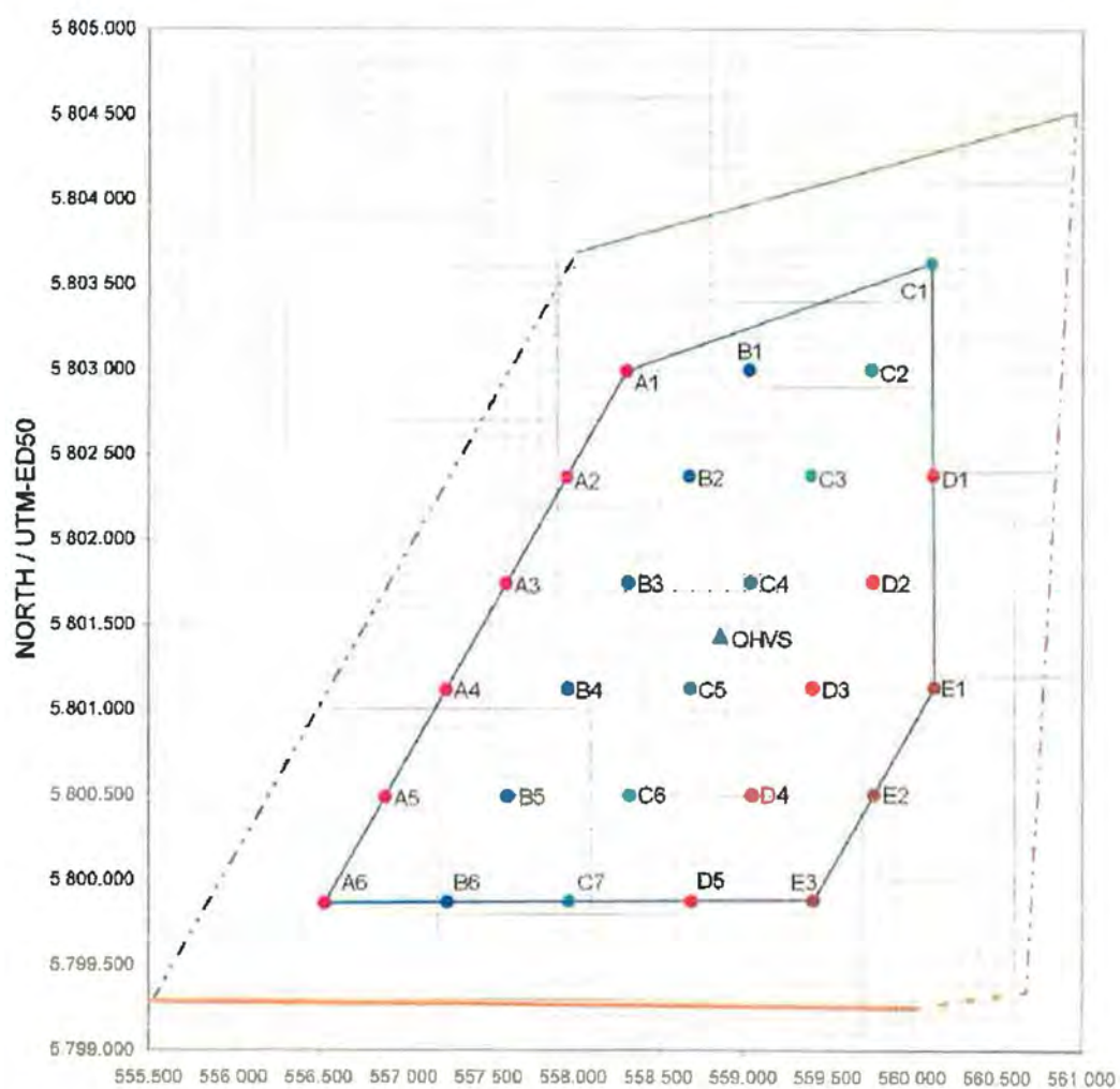
Figuur S.6 Inrichting offshore windpark Rijnveld Noord/Oost 4,5 MW compacte variant
