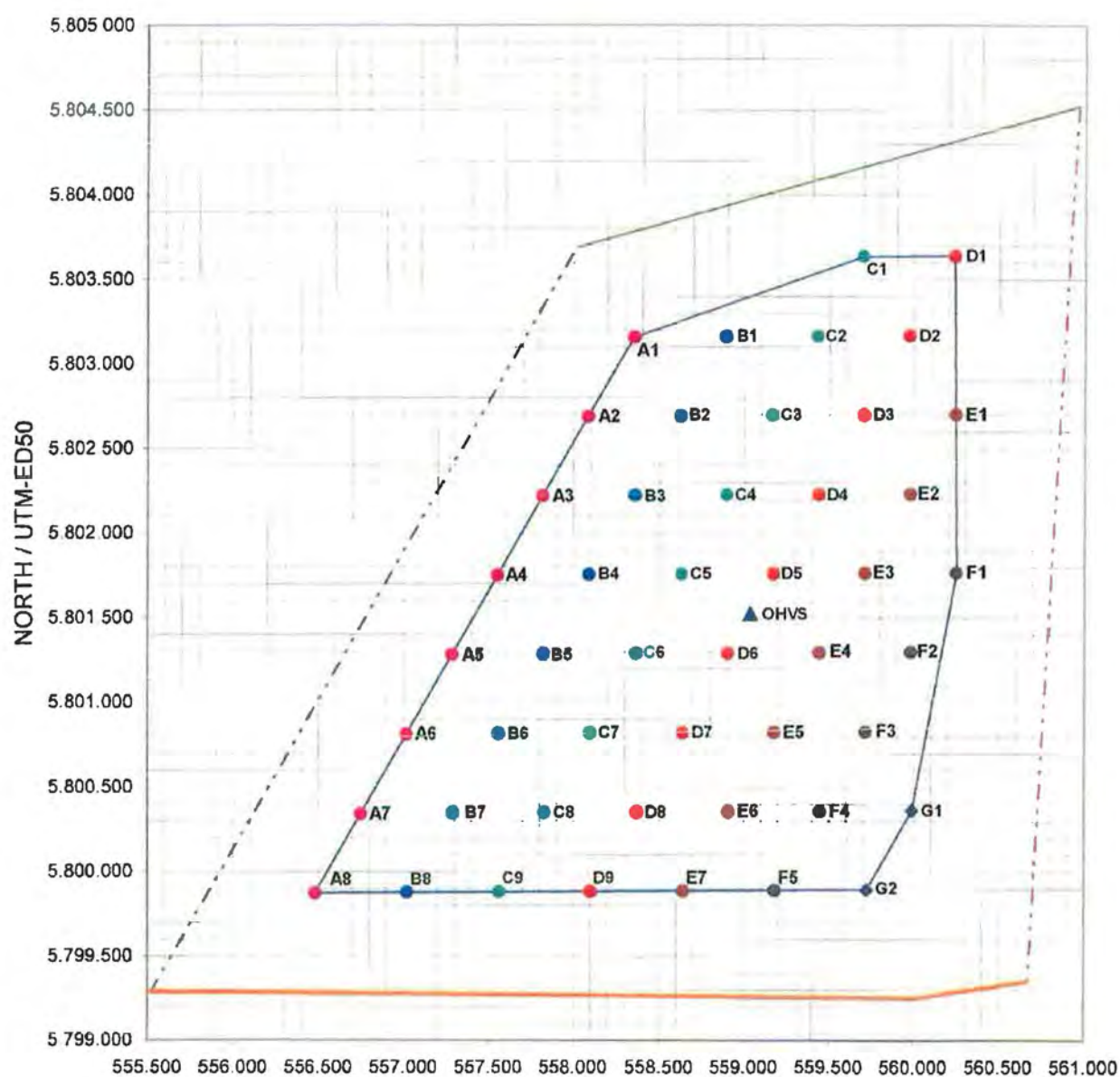
Figuur S.4 Inrichting offshore windpark Rijnveld Noord/Oost 3 MW compacte variant
