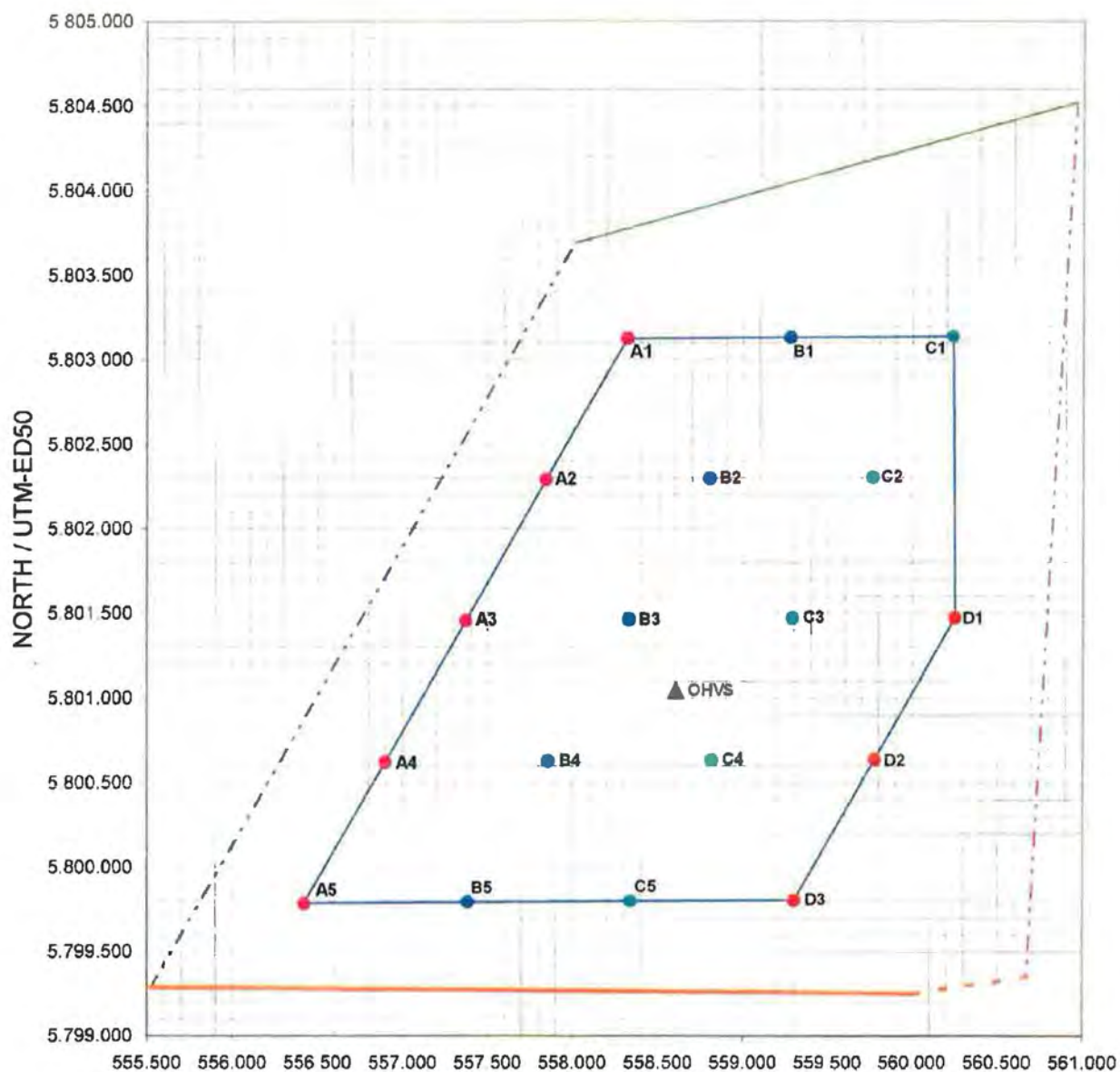
Figuur S.5 Inrichting offshore windpark Rijnveld Noord/Oost 4,5 MW basisvariant
