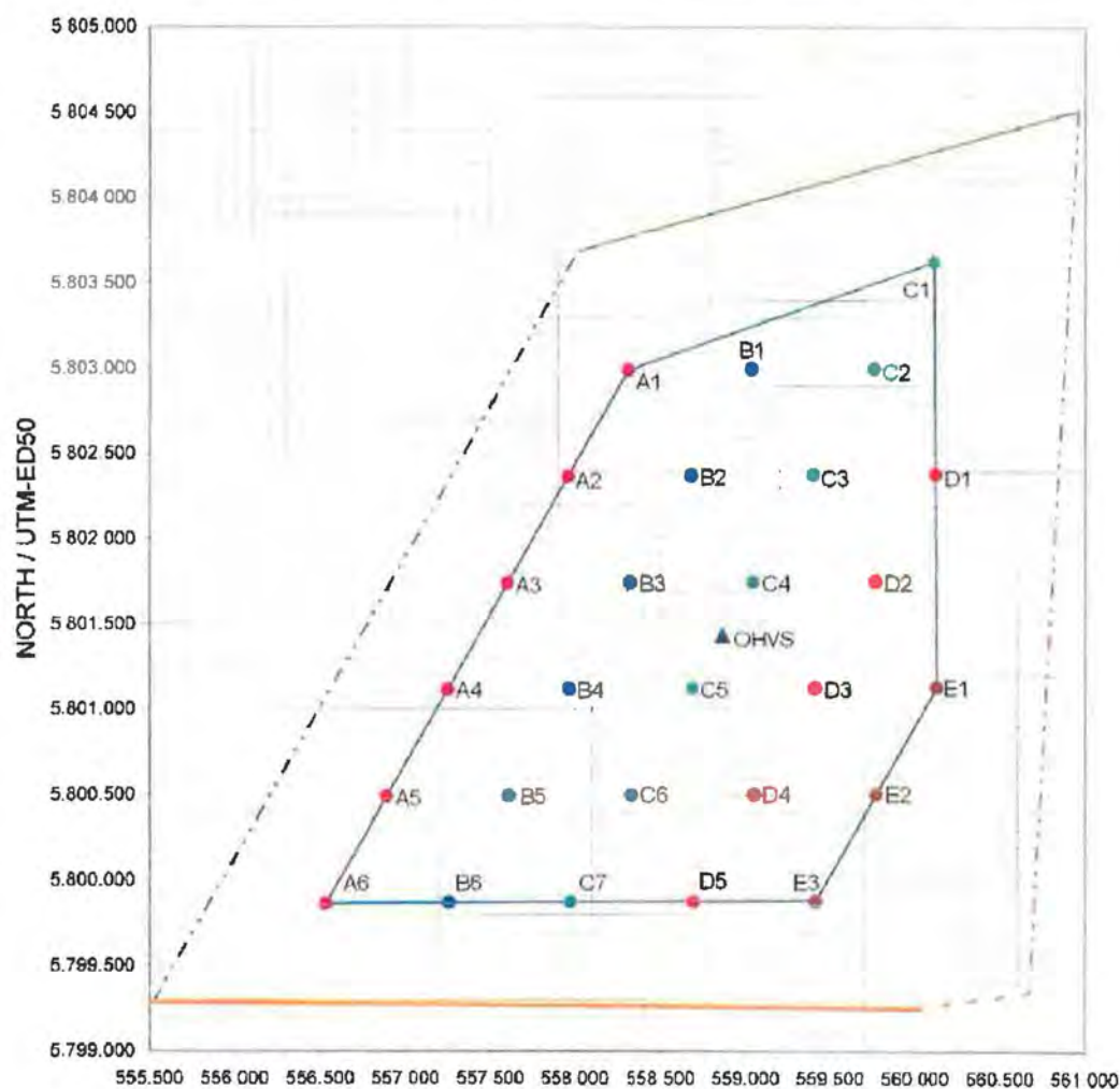
Figuur S.3 Inrichting offshore Windpark Rijnveld Noord/Oost – 3 MW – basisvariant
