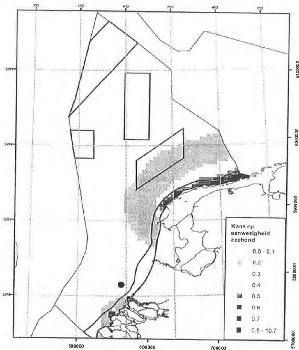
Figuur 10A.4 Berekende kans op aanwezigheid van zeehonden, gebaseerd op zwemgedrag van zeven gezenderde zeehonden [Lindeboom et al. 2005]
