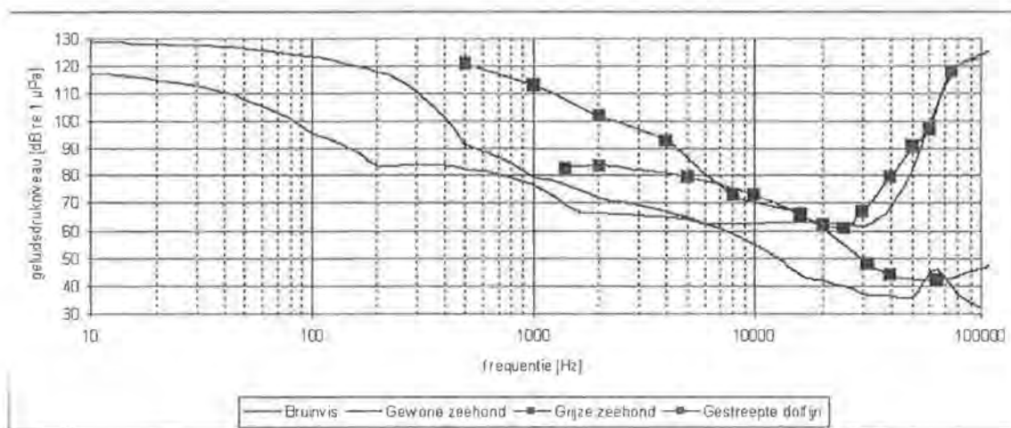
Figuur 10A.5 Audiogram van verschillende soorten met omringend geluid als referentie
