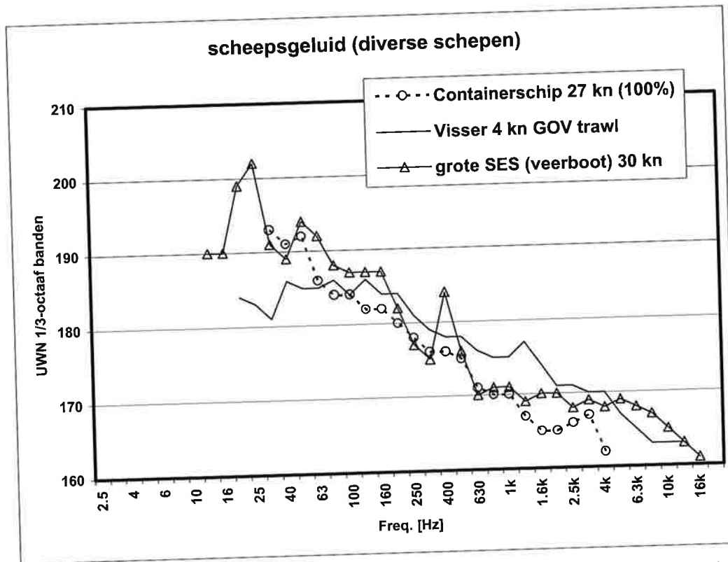
Figuur 25: de gemiddelde bronniveaus ( L_{eq} ) van diverse schepen, gemeten in 1/3-octaf bandbreedte en in dB re 1 \cdot \text{Pa}^2 \text{ m}^2 .
