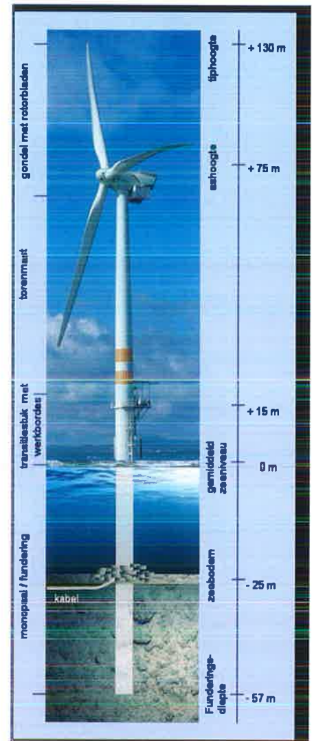
Figuur 3: opbouw van de windturbine (3,6 MW)
