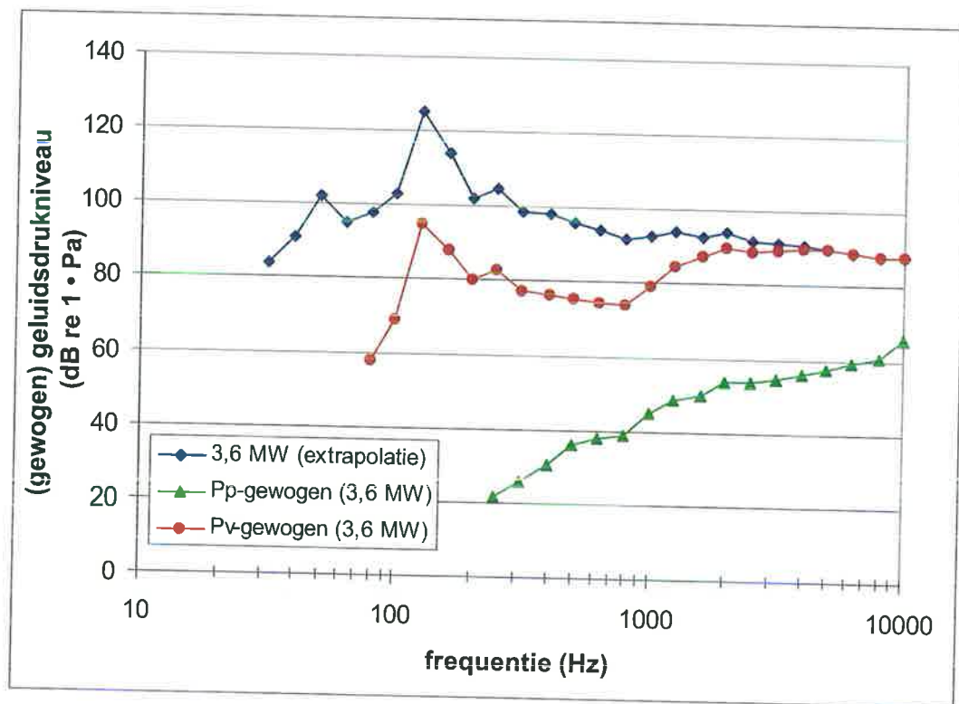
Figuur 16: op metingen in het windpark Paludans Flak gebaseerde ongewogen en audiogram gewogen geluidsspectra op 100 m van de windturbine; frequentie in tertsbanden; Pp = Bruinvis ( Phocoena phocoena ); Pv = Gewone zeehond ( Phoca vitulina )
