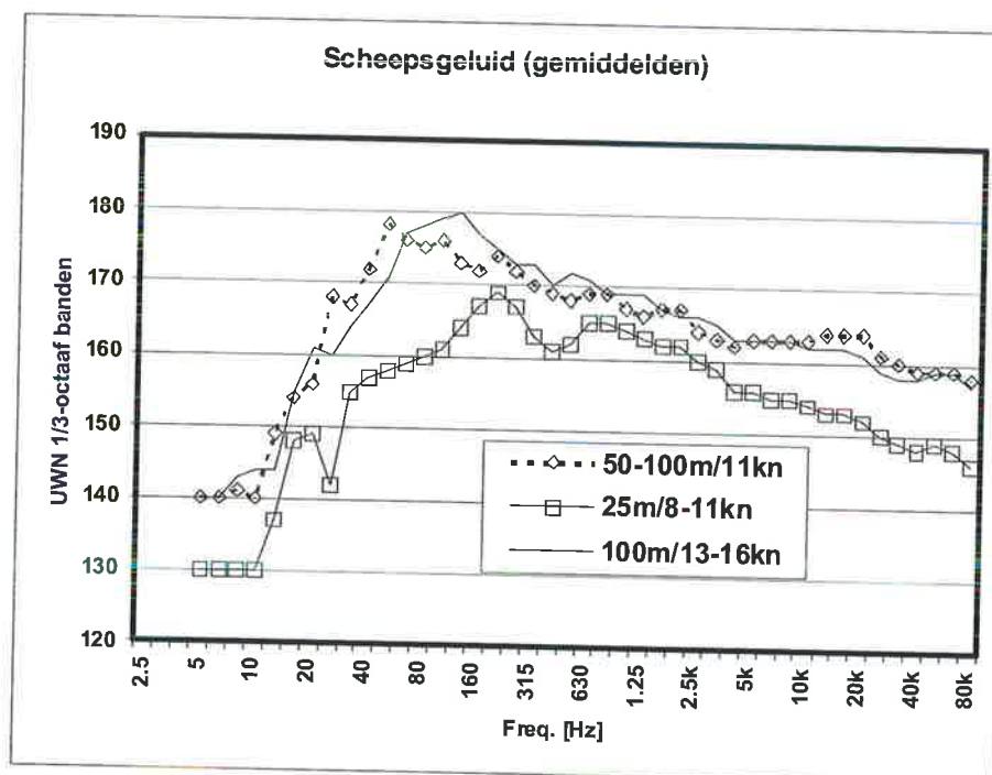
Figuur 24: de gemiddelde bronniveaus ( L_{eq} ) van diverse schepen, gemeten volgens militaire standaards, in 1/3-octaf bandbreedte en in \text{dB re } 1 \cdot \text{Pa}^2 \text{ m}^2 .
