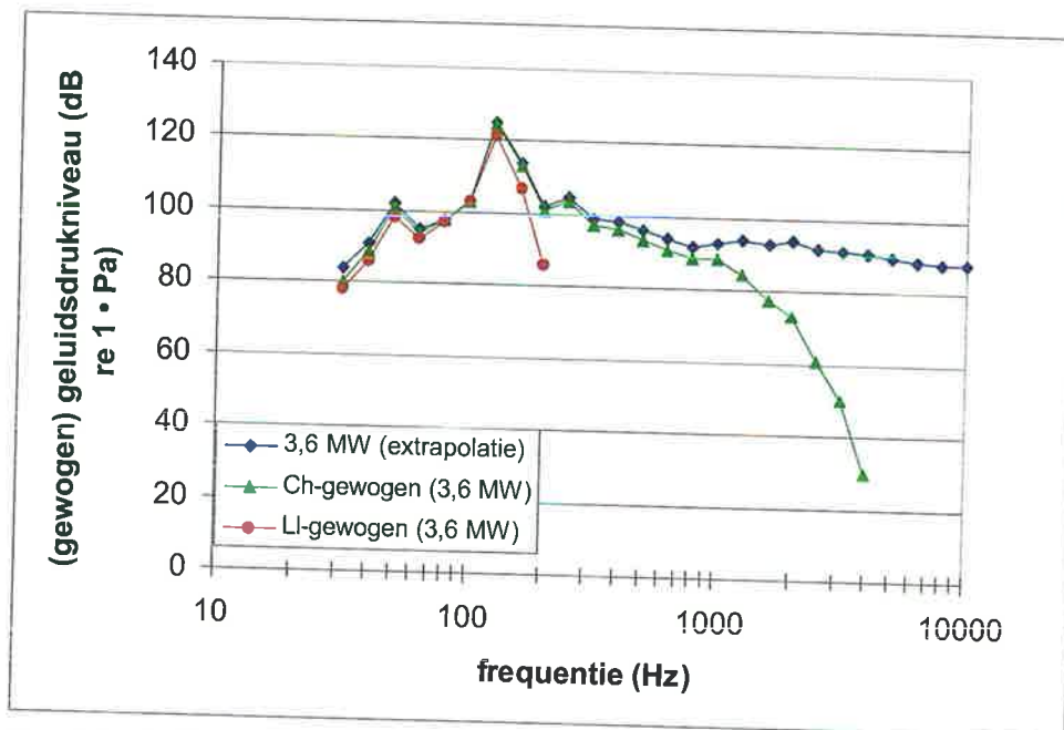
Figuur 17: op metingen in het windturbinepark Paludans Flak gebaseerde ongewogen en audiogram gewogen geluidsdruk-niveaus in tertsbanden op 100 m van de windturbine; Ch = Haring ( Clupea harengus ); LI = schar ( Limanda limanda )
