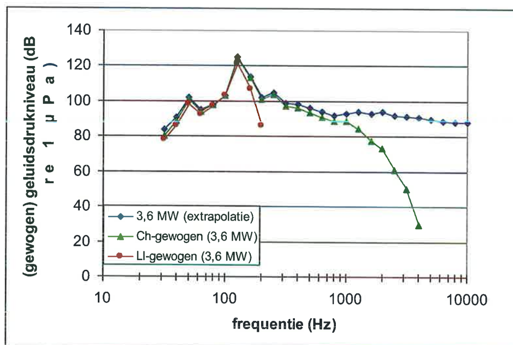
Figuur 17: op metingen in het windturbinepark Paludans Flak gebaseerde ongewogen en audiogram gewogen geluidsdrumniveaus in tertsbanden op 100 m van de windturbine; Ch = Haring ( Clupea harengus ); LI = schar ( Limanda limanda )
