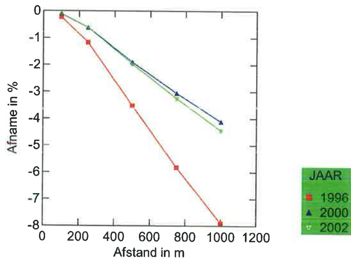
Figuur 18: afname in aantal larven (in % t.o.v. de referentie) als functie van de afstand waarover sterfte door heien optreedt.
