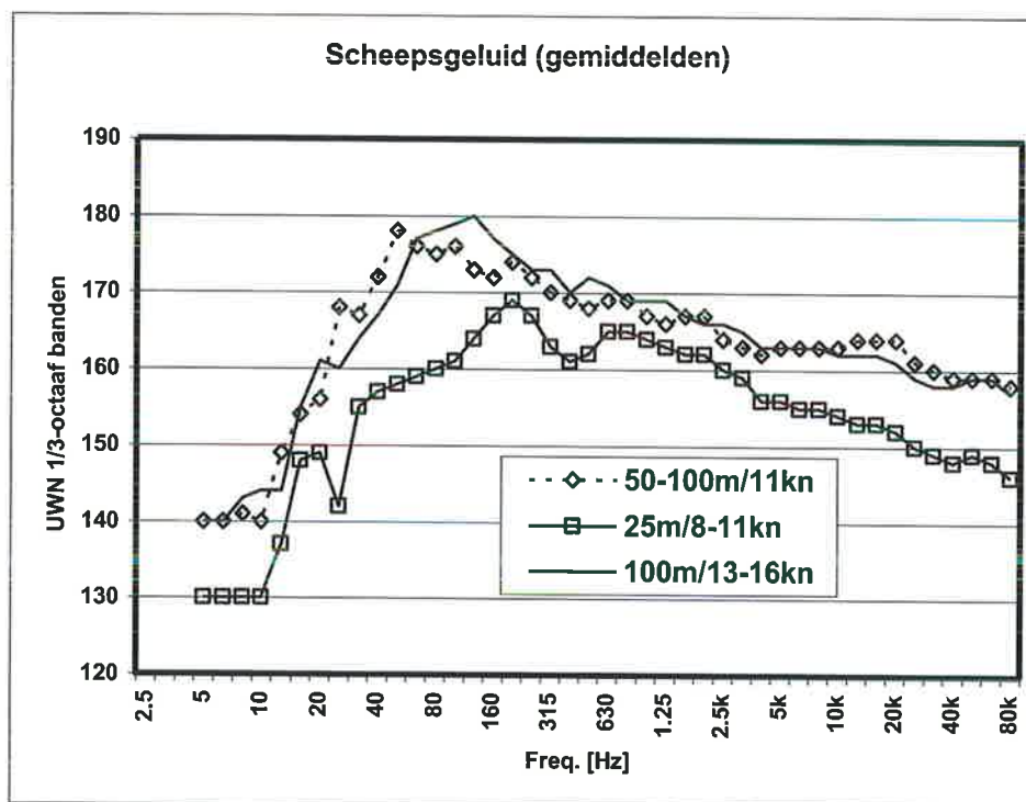
Figuur 26: de gemiddelde bronniveaus ( L_{eq} ) van diverse schepen, gemeten volgens militaire standaards, in 1/3-octaf bandbreedte en in dB re 1 \mu Pa^2 m^2 .
