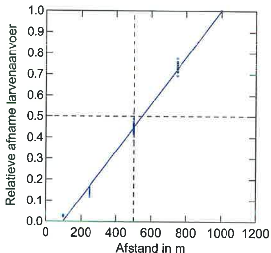
Figuur 19: relatief effect van de afstand waarover sterfte door heien optreedt op de afname van het aantal larven. Bij y=0 is er geen afname van het aantal larven, bij y=1 is de afname van het aantal larven gelijk aan de afname bij een effectafstand van 1000 m.
