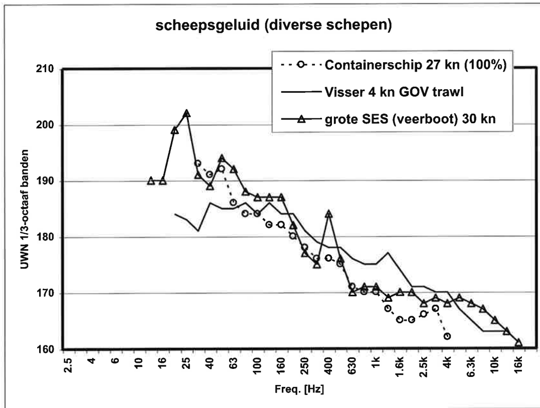
Figuur 27: de gemiddelde bronniveaus ( L_{eq} ) van diverse schepen, gemeten in 1/3-octave bandbreedte en in dB re 1 \mu\text{Pa}^2 \text{ m}^2 .
