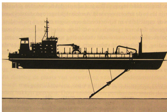
Figuur 5.1: Sleephopperzuiger
