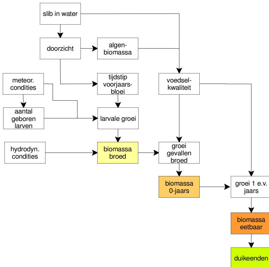
Figuur 7.2: Effectketen tussen slibconcentraties en schelpdieretende duikeenden
