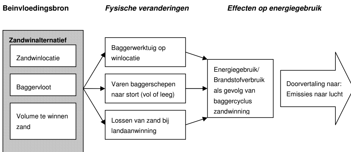
Figuur 8.1: Ingreep-effectketen energiegebruik zandwinning
