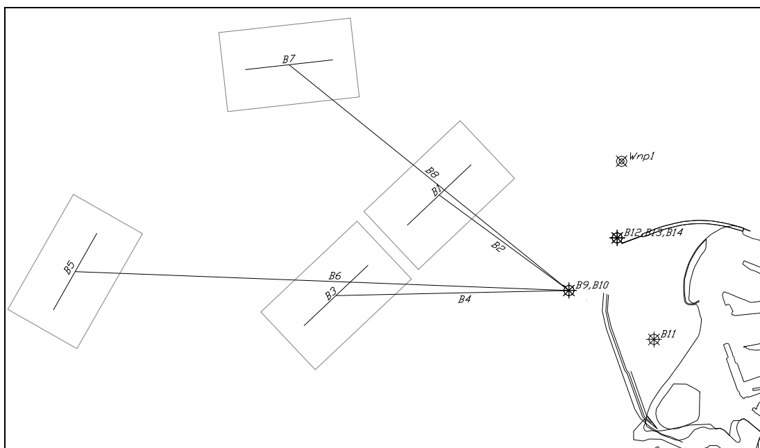
Figuur 3: Ligging geluidsbronnen zandwinning en aanleg in het rekenmodel voor peilmoment M2
