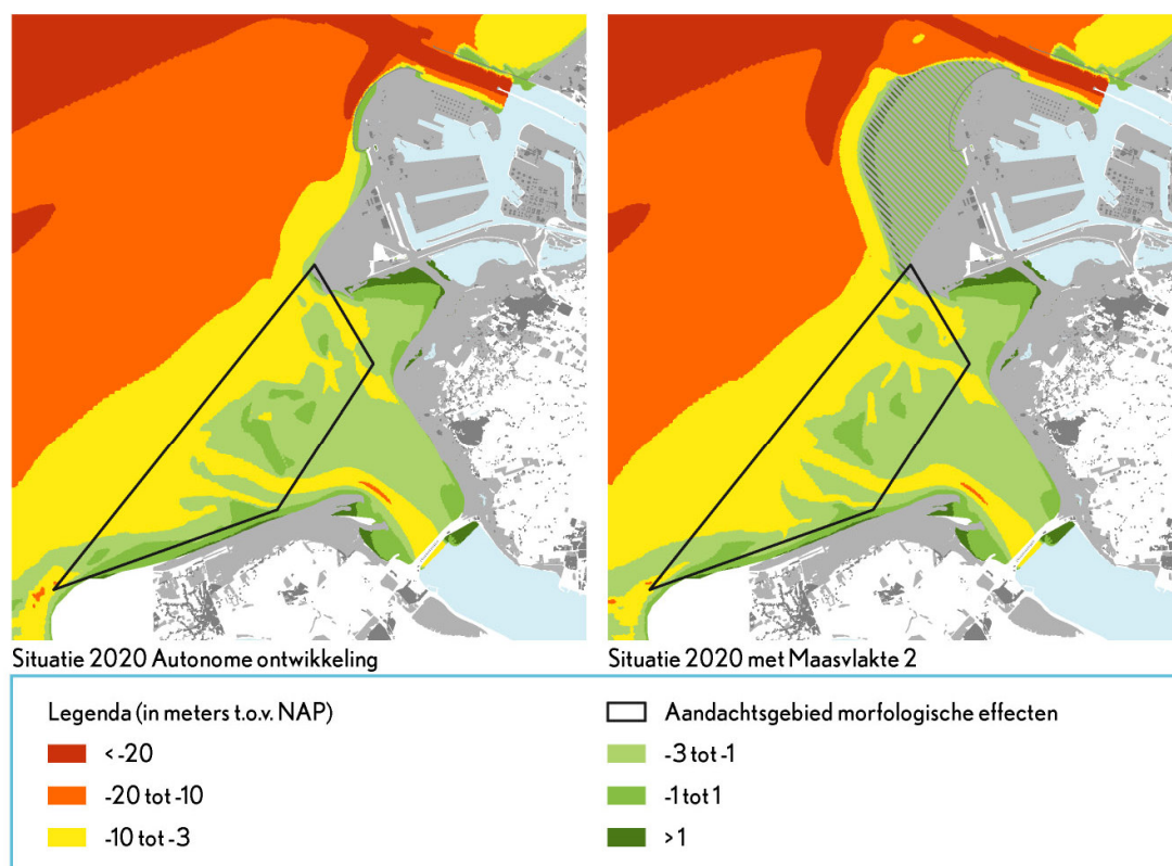
Figuur B1.4: De voorspelde morfologische situatie in de Haringvlietmonding zonder Maasvlakte 2 (links) en met Maasvlakte 2
