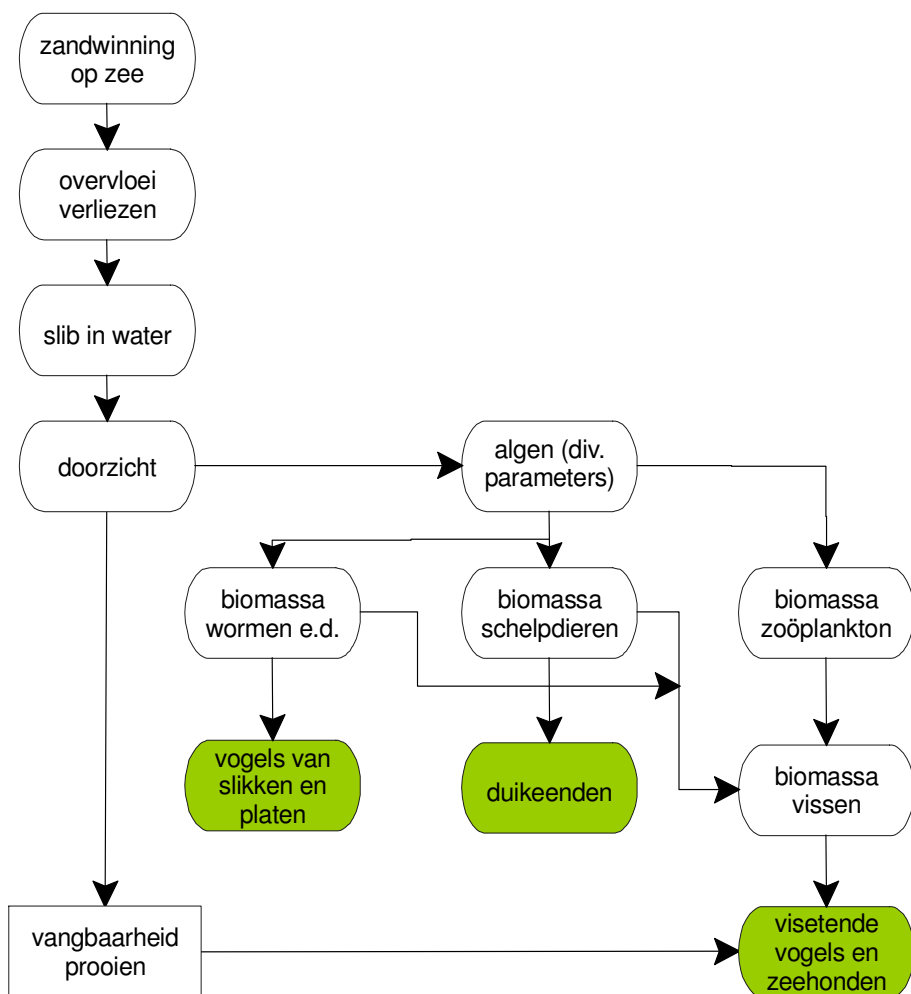
Figuur B5.3 Relaties tussen ingreep (zandwinning op de Noordzee) en effecten op soortgroepen van beschermde soorten (groen) in de Voordelta. Factoren die niet door de zandwinning worden beïnvloed zijn niet in het schema opgenomen.
