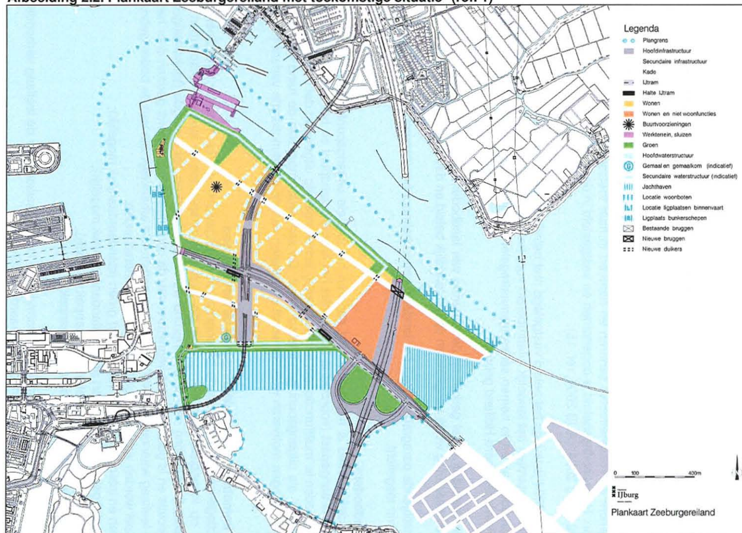
Afbeelding 2.2. Plankaart Zeeburgereiland met toekomstige situatie* (ref. 1)
