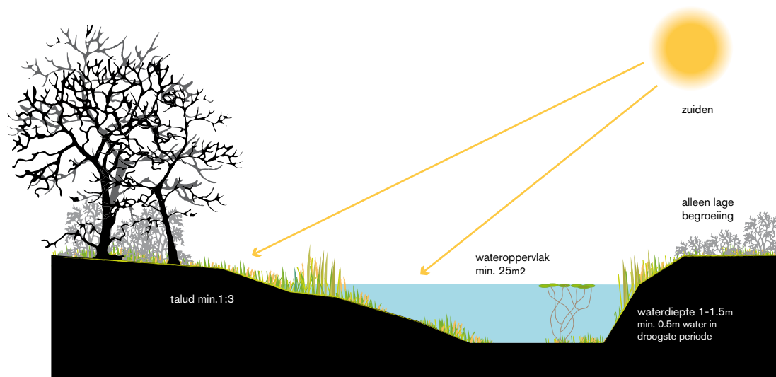
Schematische weergave van een goede poel (principe profiel)
