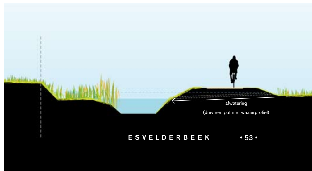
Detail profiel waterafvoer
