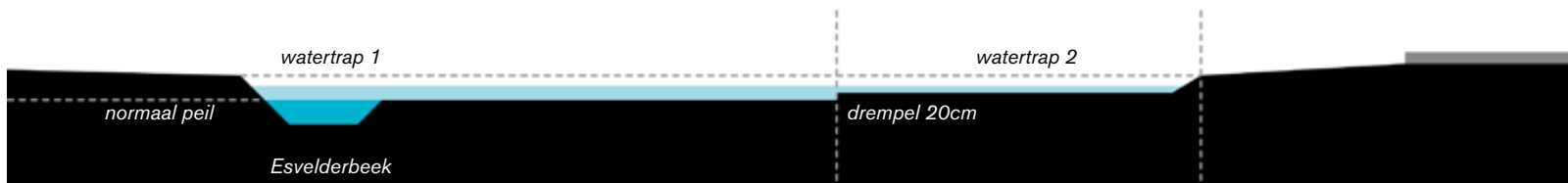
'getrapte overloop' (Actualisatie WSP, gem. Barneveld): watertrap 1: 0.20m peilstijging, watertrap 2: 0.40m peilstijging
