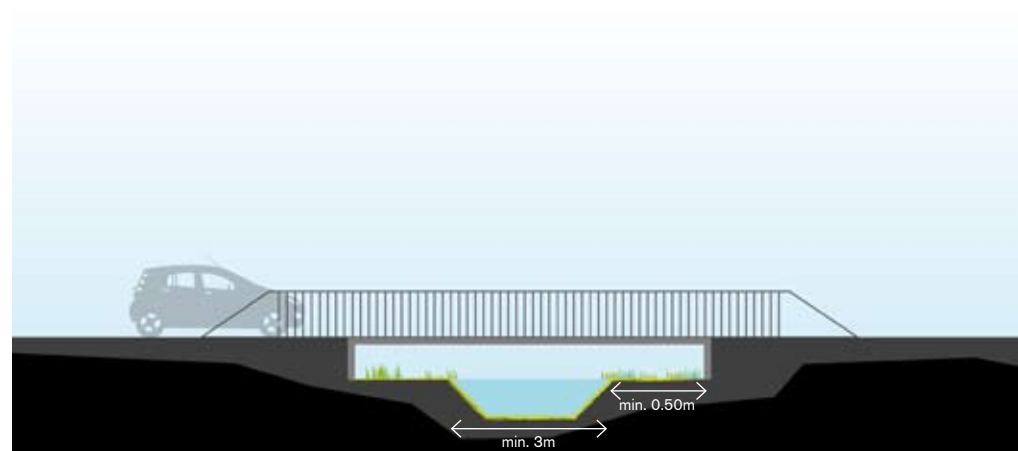
Profiel flora- en fauna passage
