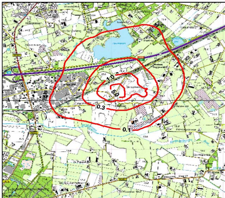
Figuur 12.3 Bijdrage Vink afvalverwerking aan PM_{10} -concentraties in 2007 ( \mu g/m^3 als jaargemiddelde)
