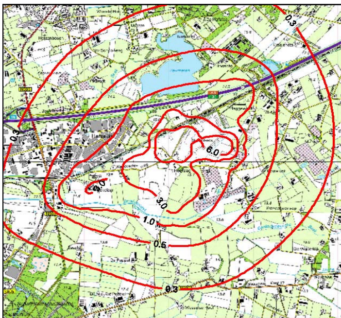
Figuur 12.5 Bijdragen industriële bronnen aan PM 10 -concentraties in 2020 (µg/m 3 als jaargemiddelde)
