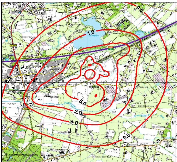
Figuur 12.4 Bijdragen industriële bronnen aan NO 2 -concentraties in 2020 (µg/m 3 als jaargemiddelde)
