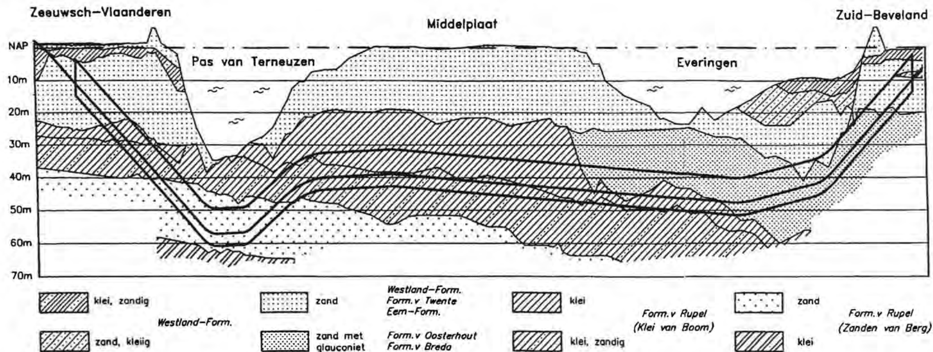
Figuur 2-2 Geologische profiel Tunneltracé
