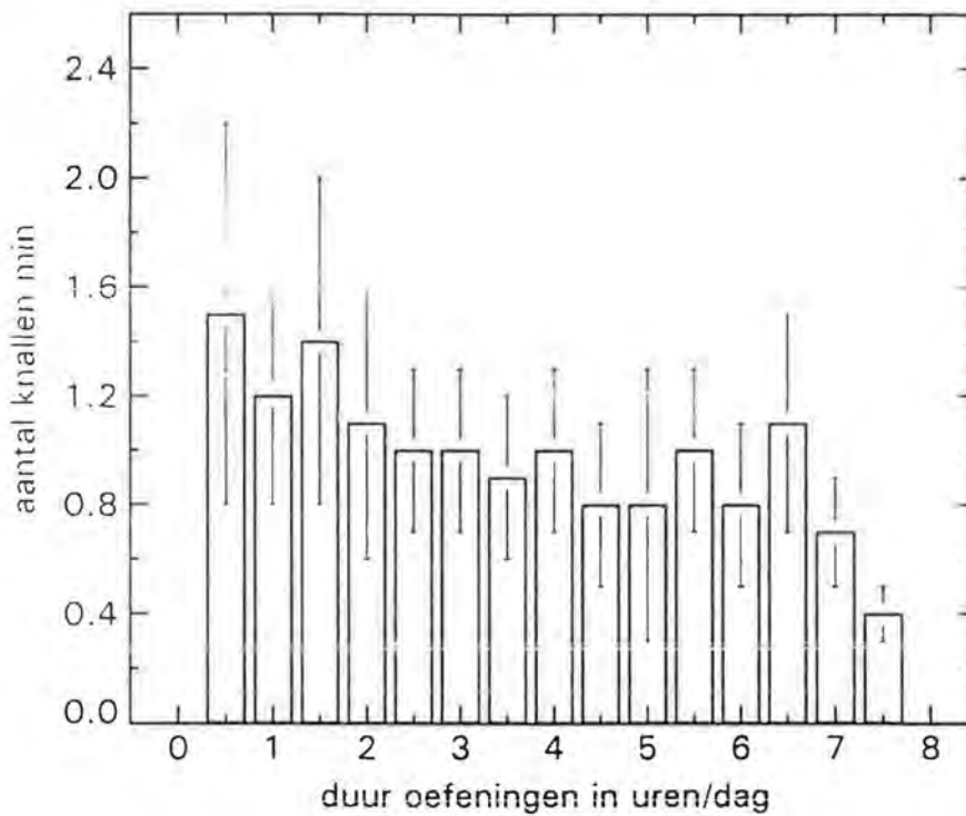
Fig. 4 Munitieverbruik in aantal handgranaten per minuut als functie van de duur van de oefeningen. De verticale lijnen geven de standaarddeviatie om het gemiddelde weer.
