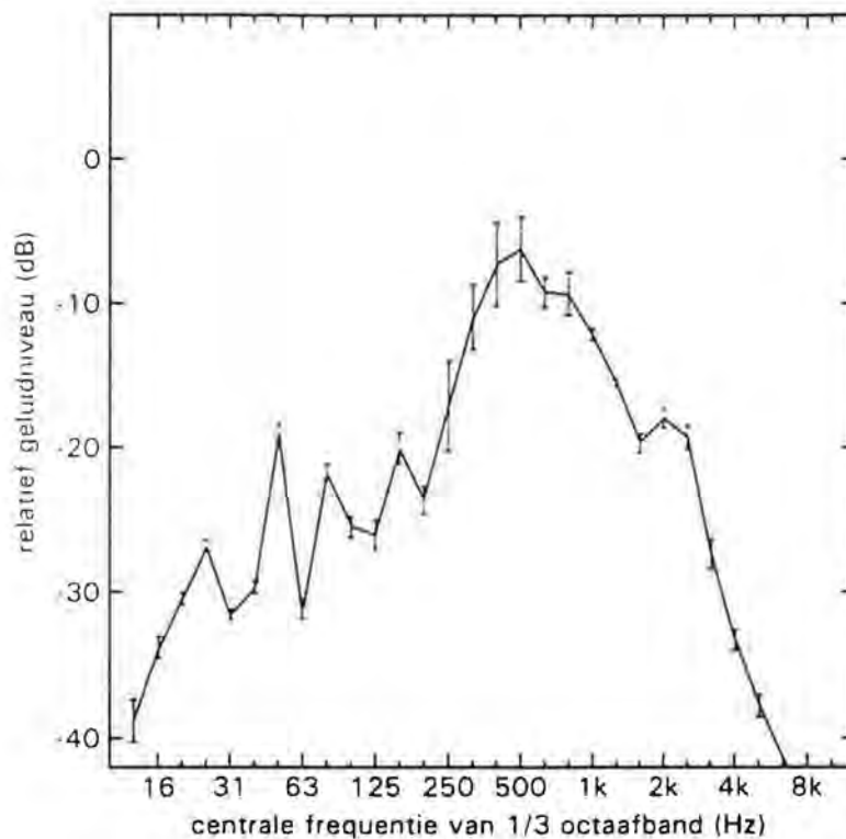
Fig. 12 Gemiddeld spectrum in 1/3-octaaftanden voor de met lichte vuurwapens geproduceerde knallen. De over diverse perioden van 30 s bepaalde equivalente geluidsdruk-niveaus per 1/3-octaaftand worden gegeven ten opzichte van het overall lineaire equivalente geluidsdruk-niveau. De verticale lijnen geven de standaarddeviatie van het gemiddelde weer.
