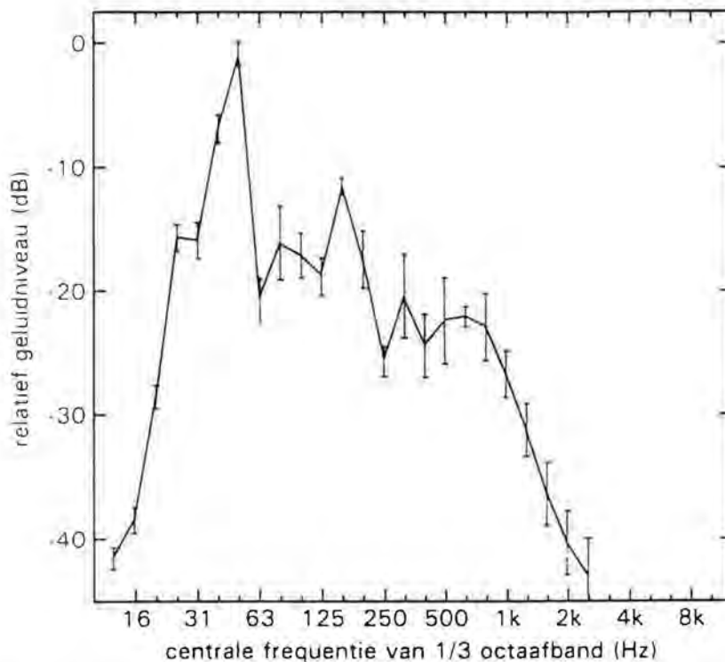
Fig. 7 Gemiddeld spectrum in 1/3-octaaftanden voor de knallen van detonerende handgranaten. De 1/3-octaaftniveaus worden gegeven ten opzichte van het maximum overall niveau in dB(lin,fast). De verticale lijnen geven de standaarddeviatie om het gemiddelde weer.
