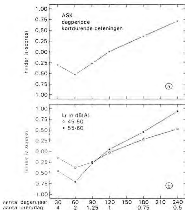
Fig. 24 Verwachte hinder ten gevolge van schietoefeningen in de dagperiode, voor (a) de gematigd en zwaarder belaste groep respondenten samen, en (b) de beide groepen afzonderlijk.
