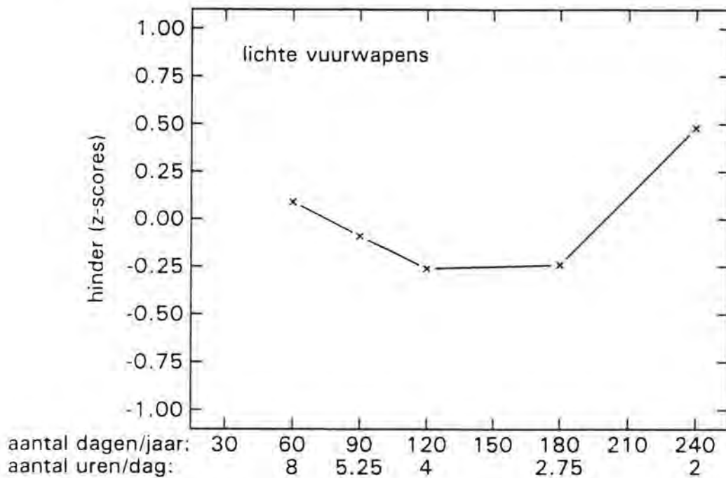
Fig. 13 Hinderscores ten gevolge van oefeningen met lichte vuurwapens, als functie van het aantal oefendagen per jaar.
