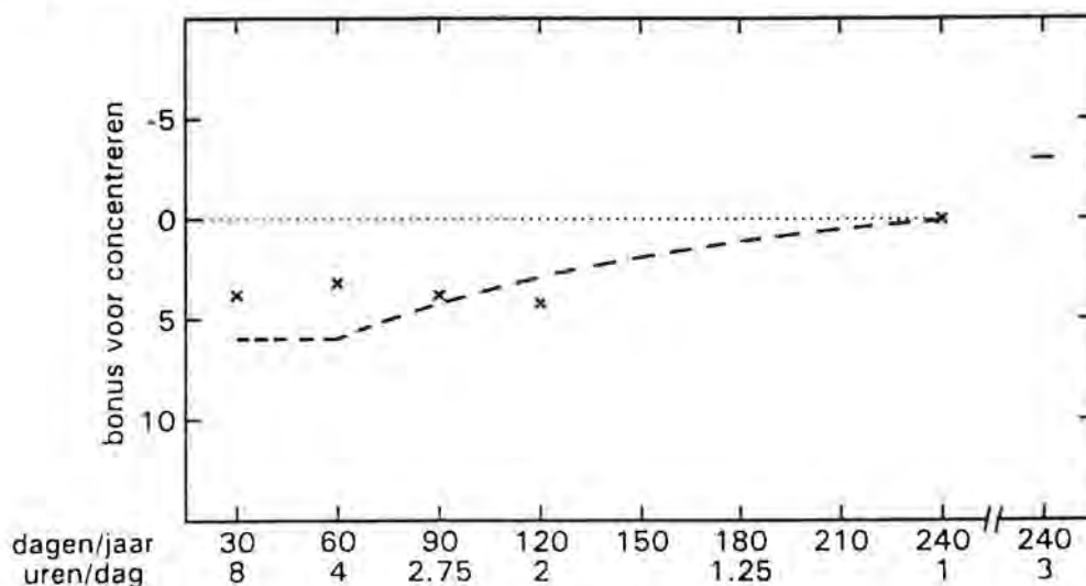
Fig. 34 De bonus waarmee L_r volgens een Zwitserse procedure mag worden verminderd, voor de scenario's die ook in Fig. 33 zijn beschreven. De bonus voor de diverse scenario's is uitgedrukt ten opzichte van het scenario met 240 1-urige schietdagen. De kruisjes zijn resultaten die zijn verkregen in het in § 8.2 beschreven experiment.
