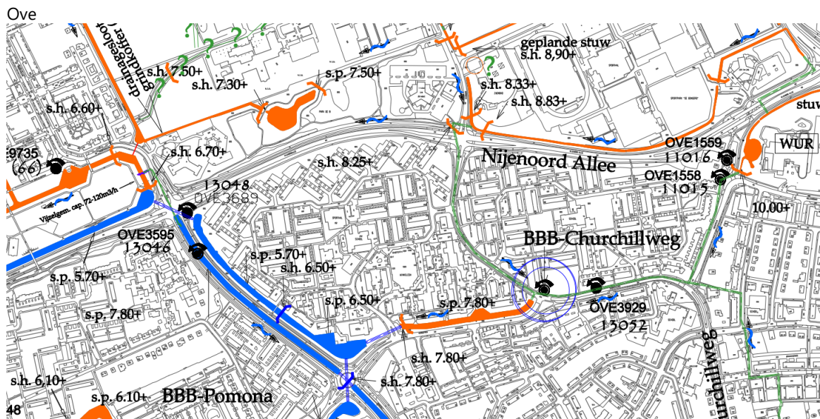
Afbeelding 2.3 Overzicht van de peilregulerende kunstwerken + gehanteerde peilen. (bron: STUW-overzicht Wageningen_2012)
