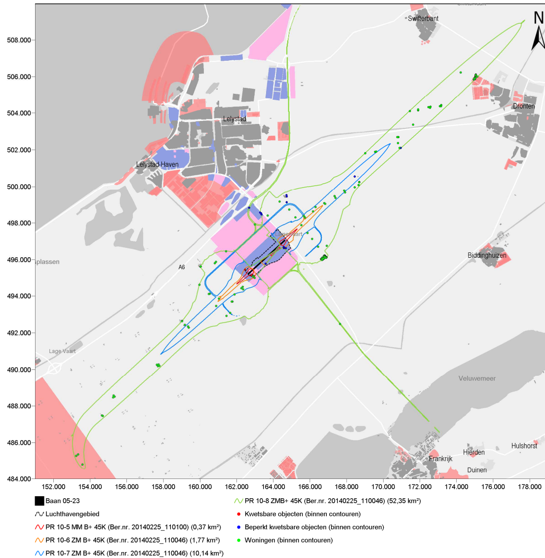
Figuur 20 PR-contouren voor het 45k scenario routevariant B+.
