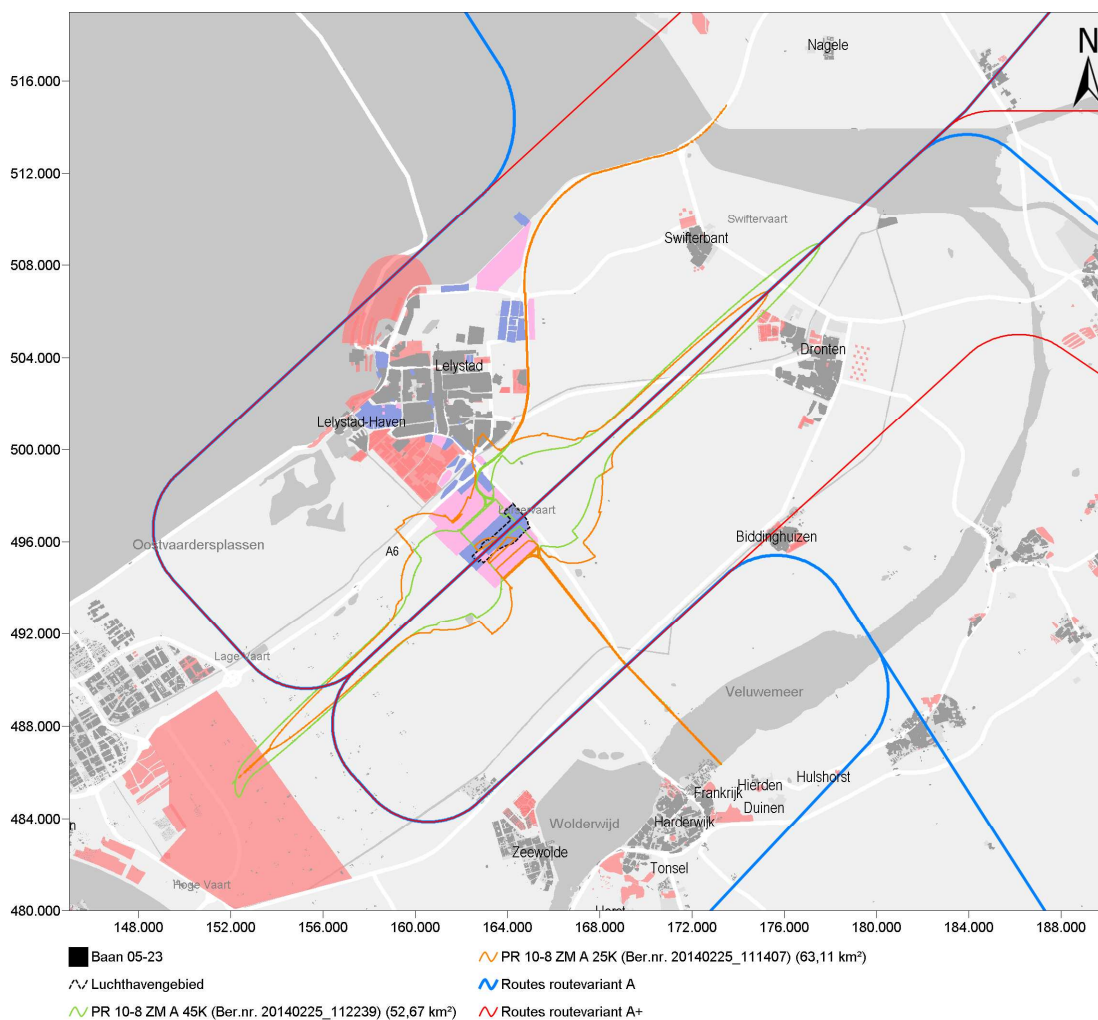
Figuur 11 10^{-8} PR-contouren voor routevariant A met daarbij de routes voor variant A en A+ weergegeven.
