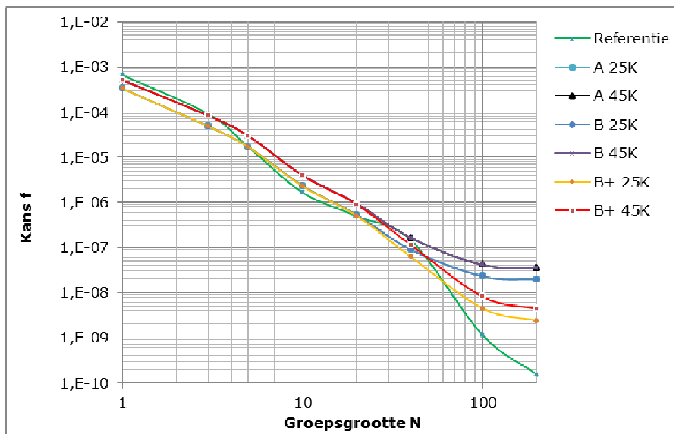
Figuur 12 Vergelijking FN-curves voor referentie en de routevarianten voor de voorgenoemde activiteit.
