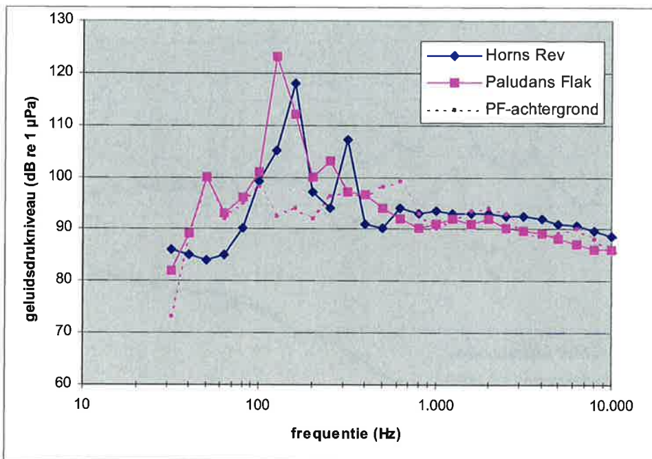
Figuur 18: in twee windparken gemeten, in tertsbanden weergegeven geluidsspectra; metingen op circa 100 m van de windturbine (naar ISD, 2007); zie ook Tabel 16; de gestippelde curve (PF-achtergrond) geeft het spectrum in Paludans Flak weer bij een windsnelheid van minder dan 2 m/s terwijl alle windturbines zijn uitgeschakeld.
