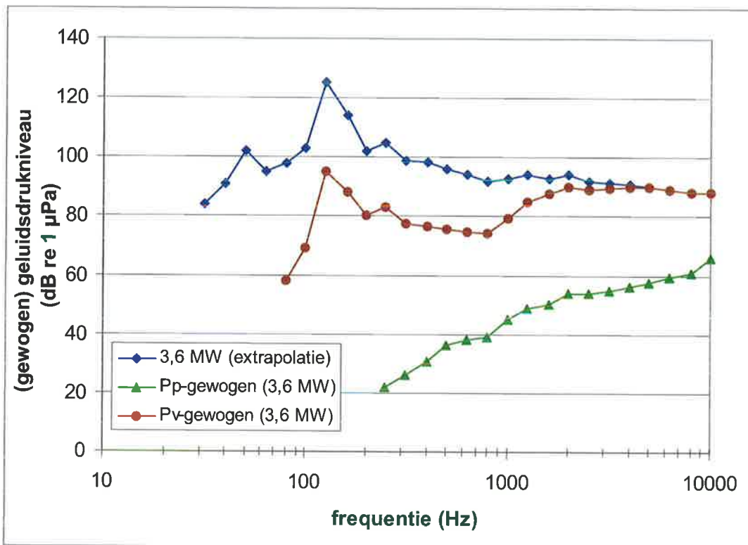
Figuur 19: op metingen in het windpark Paludans Flak gebaseerde ongewogen en audiogram gewogen geluidsspectra op 100 m van de windturbine; frequentie in tertsbanden; Pp = Bruinvis ( Phocoena phocoena ); Pv = Gewone zeehond ( Phoca vitulina )
